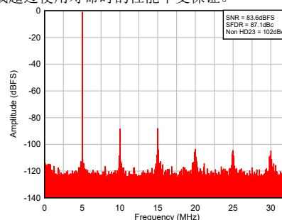
单音频谱， F_s = 65\text{MSPS} ， F_{in} = 5\text{MHz}
