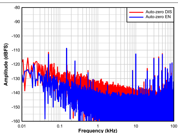
图 7-9. F_S = 10\text{MSPS} , F_{IN} = 1.1\text{MHz}
