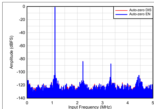
图 7-8. F_S = 10\text{MSPS} , F_{IN} = 1.1\text{MHz}
