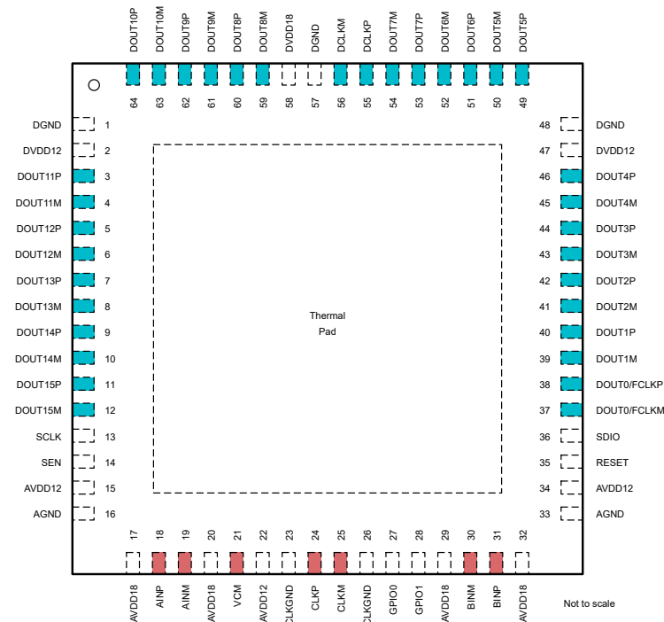
图 5-1. RTD 封装、64 引脚 VQFN (顶视图)
