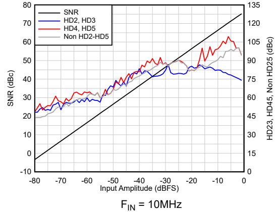
图 6-14. 交流性能与 A_{IN} 间的关系
