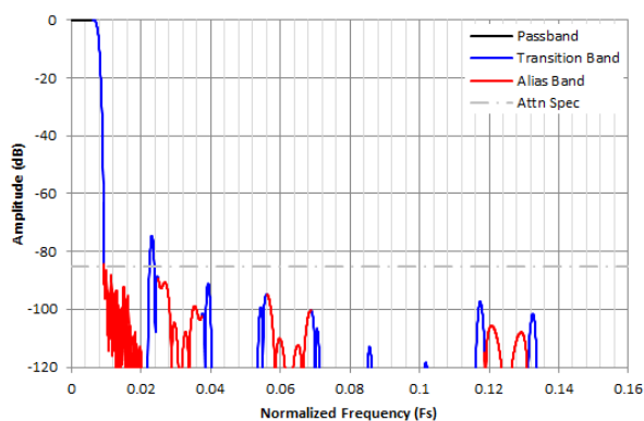
图 8-34. /64 复数抽取滤波器响应
