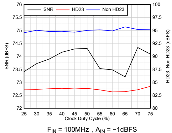
图 6-18. 交流性能与时钟占空比间的关系
