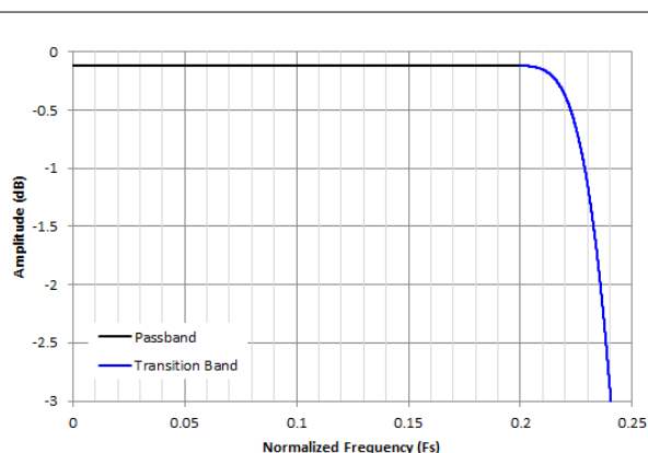
图 8-25. /2 抽取通带纹波响应
