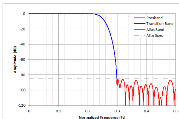
图 8-24. /2 复数抽取滤波器响应
