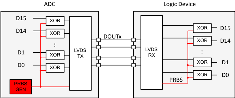
图 8-64. 输出扰频器
