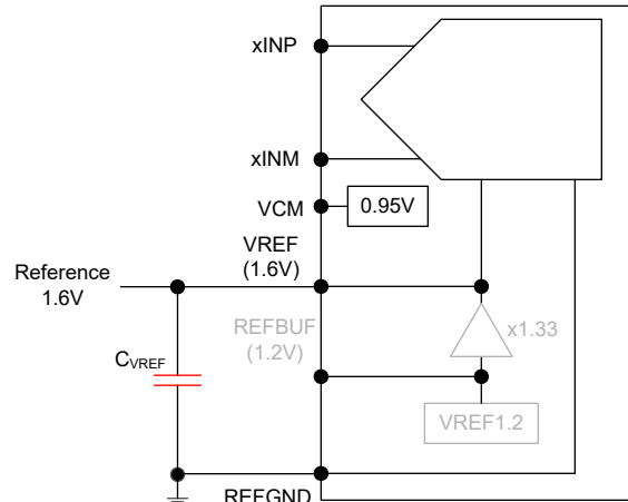
图 8-13. External 1.6V reference
