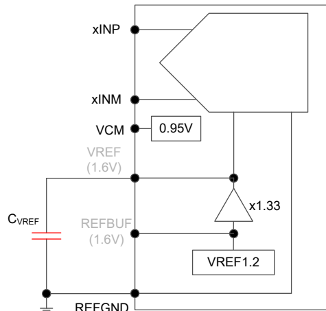
图 8-14. Internal reference
