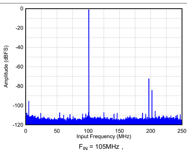
图 8-69. FFT : 低延迟模式
