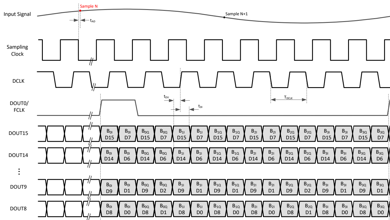
图 7-2. 时序图 - 串行 LVDS (示例：四频带、16 位、1/8 复数抽取)
