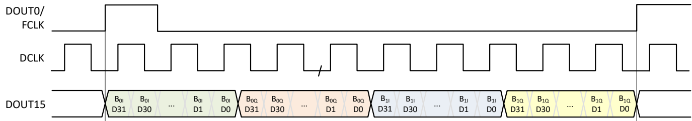
图 8-60. 示例 5 的 SLVDS 帧组装
