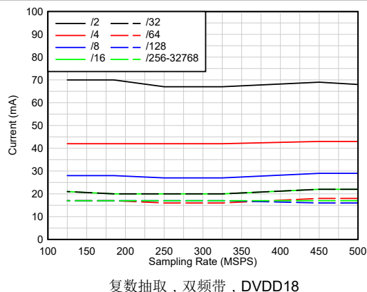
图 6-58. 电流与采样率间的关系
