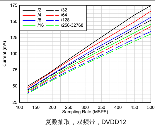
图 6-59. 电流与采样率间的关系
