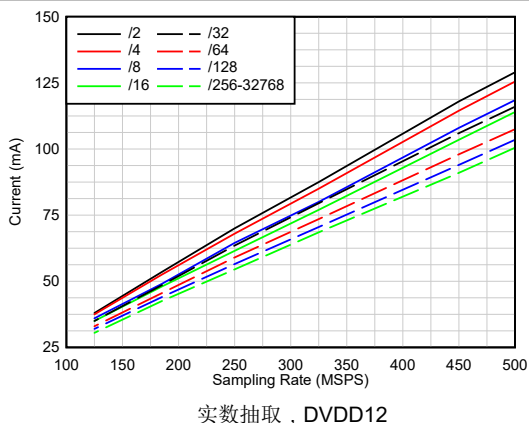
图 6-57. 电流与采样率间的关系
