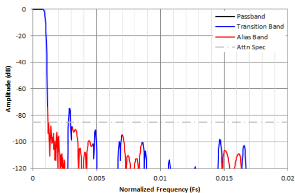
图 8-39. /512 复数抽取滤波器响应
