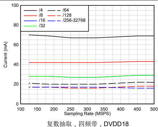
图 6-60. 电流与采样率间的关系
