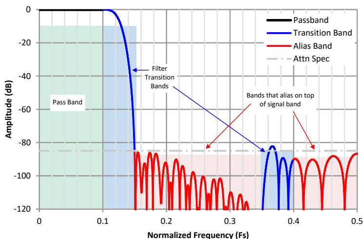
图 8-22. 抽取滤波器图的解释
