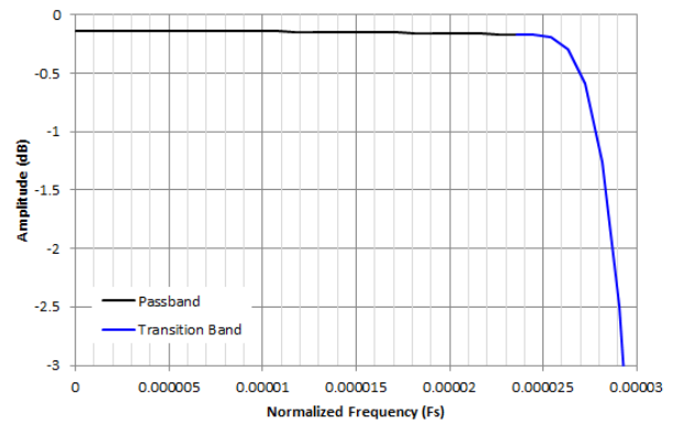
图 8-50. /16384 抽取通带纹波响应
