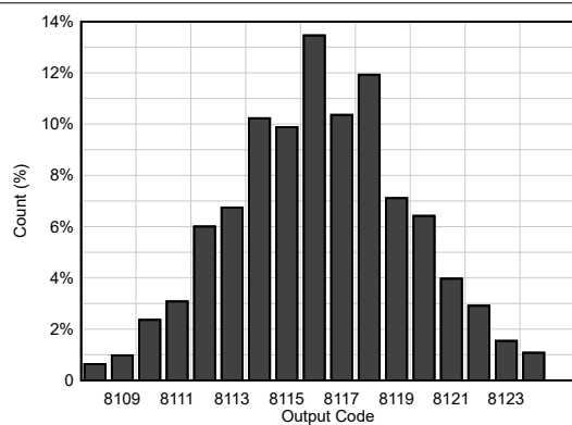
图 6-25. 直流偏移直方图
