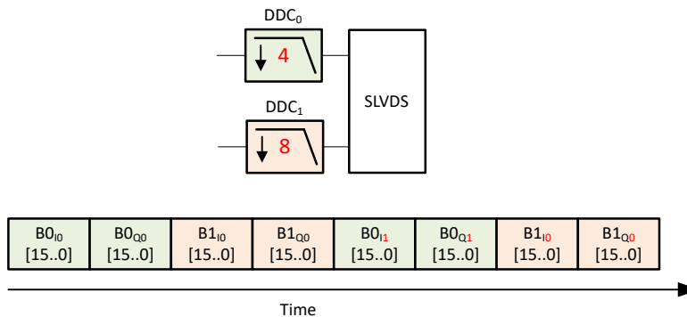
图 8-21. 不等的抽取因子
