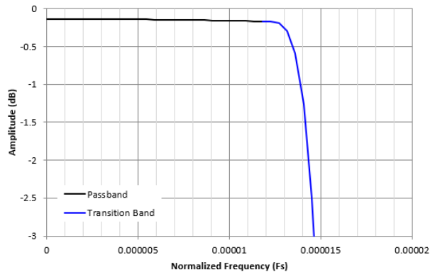
图 8-52. /32768 抽取通带纹波响应
