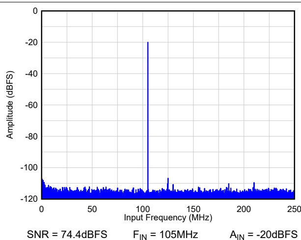
图 8-73. FFT - 无 AVG
