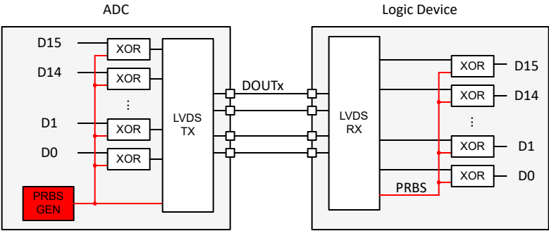
图 8-63. 输出扰频器
