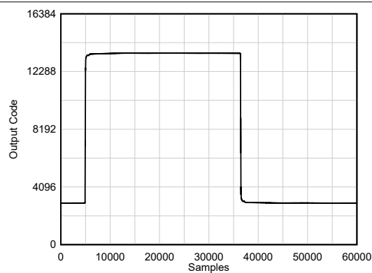
图 6-26. 脉冲响应
