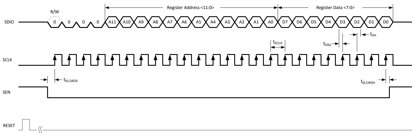
图 8-75. 串行寄存器写入时序图
