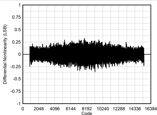
图 6-51. DNL
