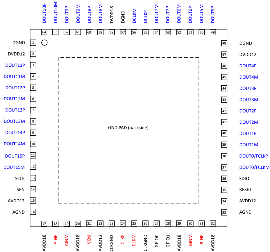
图 5-1. RTD 封装、64 引脚 VQFN (顶视图)
