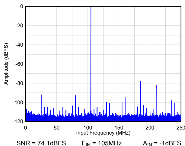
图 8-71. FFT - 无 AVG
