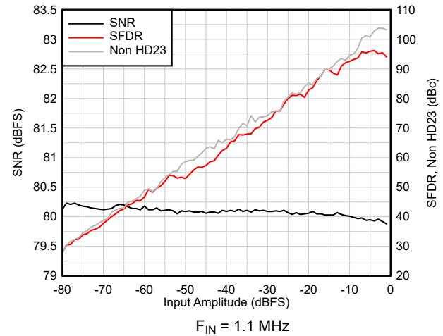
图 6-25. AC Performance vs Input Amplitude
