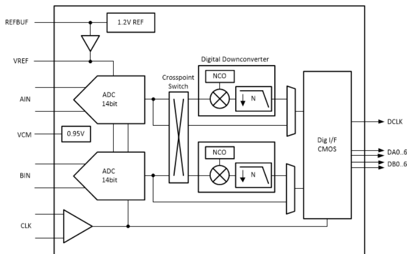
ADC364x 方框图
