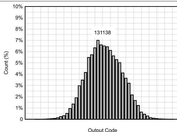
图 6-61. DC Histogram
