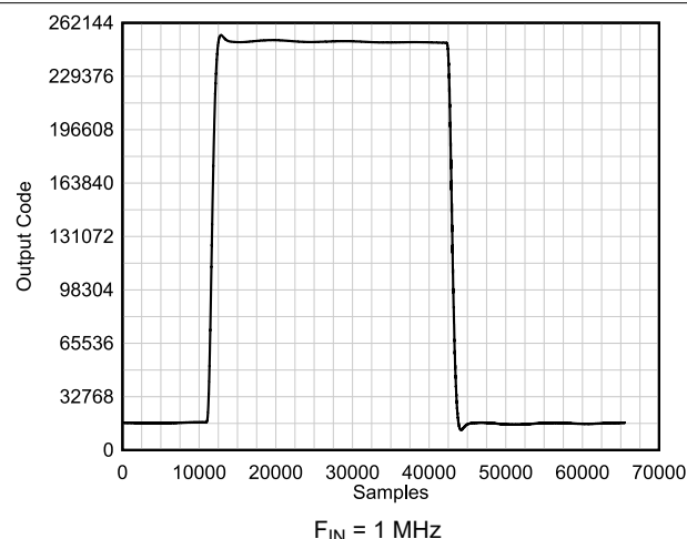
图 6-62. Pulse Response
