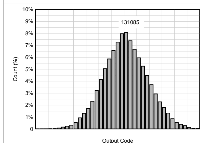
图 6-36. DC Offset Histogram
