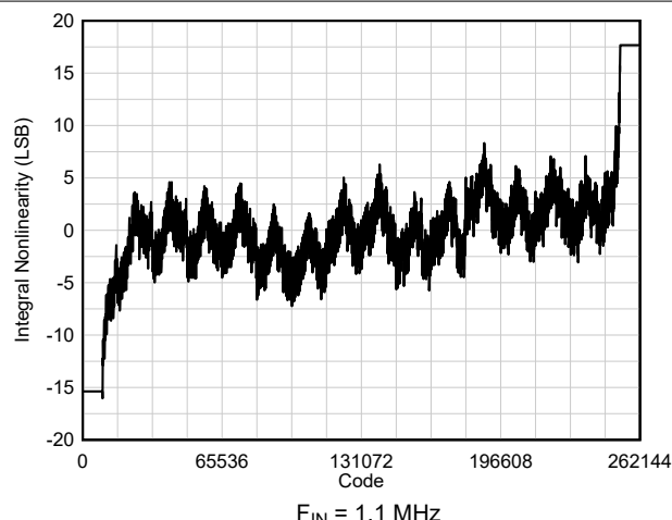
图 6-12. INL vs Code
