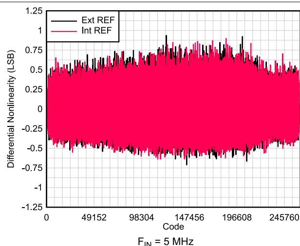
图 6-60. DNL vs Code
