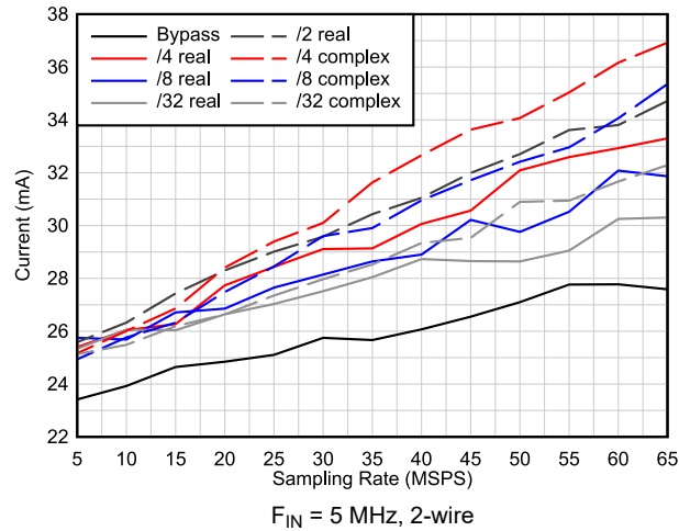
图 6-64. IOVDD Current vs Decimation
