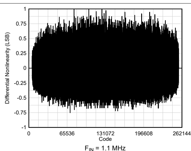
图 6-35. DNL vs Code
