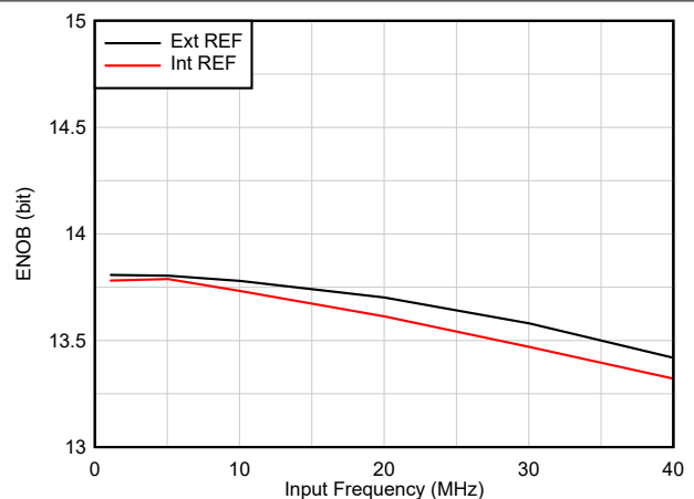
图 6-6. ENOB vs Input Frequency
