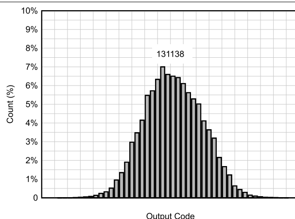
图 6-61. DC Histogram
