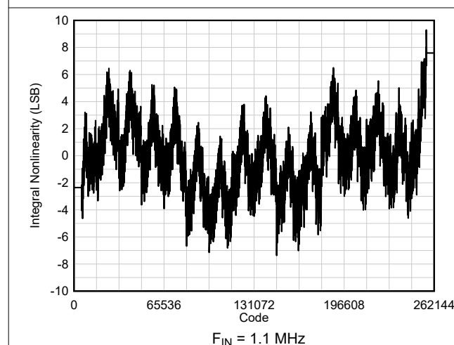
图 6-34. INL vs Code
