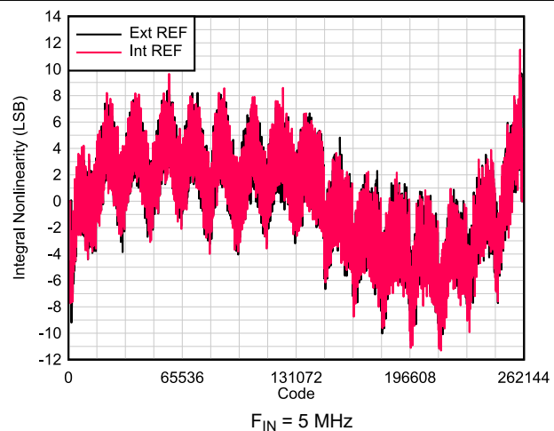
图 6-59. INL vs Code
