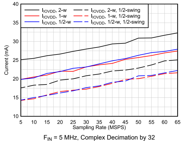
图 6-65. IOVDD Current vs Output Interface
