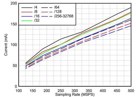
复数抽取，四频带，DVDD12
