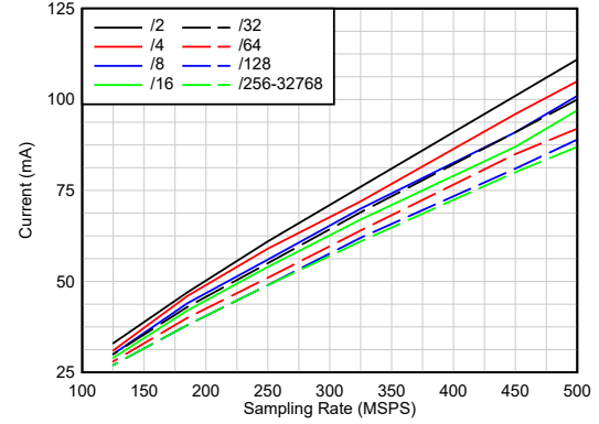
复数抽取，单频带，DVDD12
