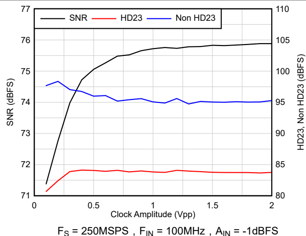
图 8-13. 交流与时钟振幅间的关系
