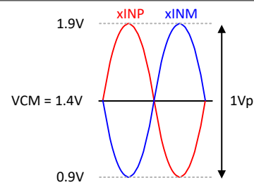
图 8-3. 模拟输入电压范围
