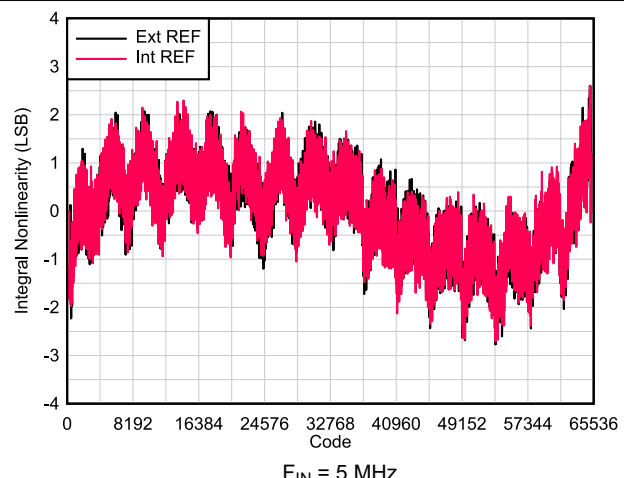
图 6-59. INL vs Code
