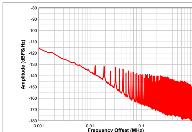
图 6-8. Dither Close-Up
