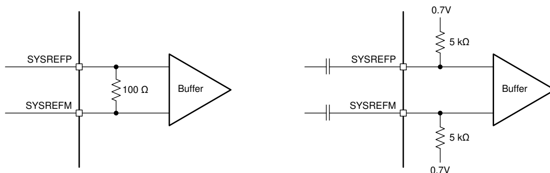
图 6-20. SYSREF Input Circuitry
