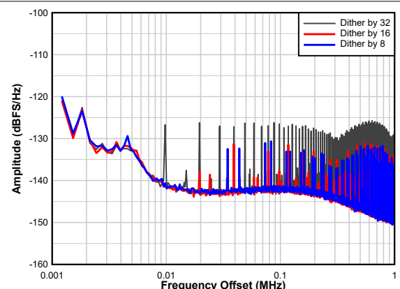
图 6-9. Dither vs Dither Divider Setting
