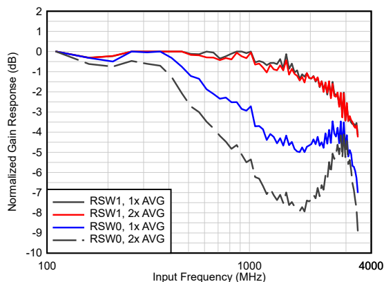
图 6-2. Input Bandwidth - Reset switch DIS
