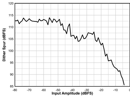
图 5-25. Dither Spur vs A_{IN}
