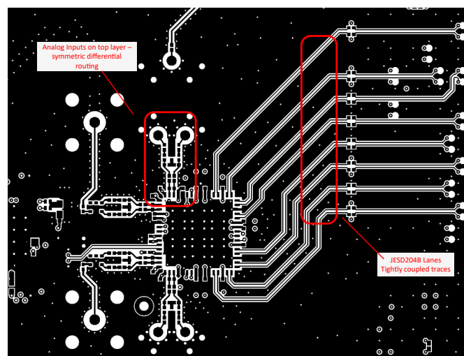
图 7-7. Layout example: top layer of ADC34RF5x EVM
