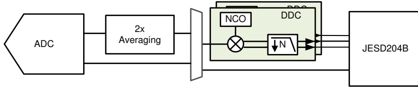
图 6-23. Digital Decimation Filter Options
