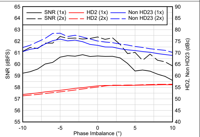
图 6-6. Phase Imbalance - 3.0 GSPS
