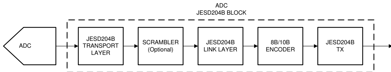
图 6-41. JESD204B Block Diagram
