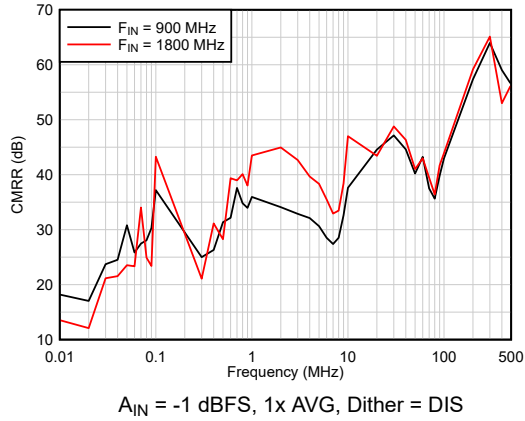
图 5-41. CMRR
