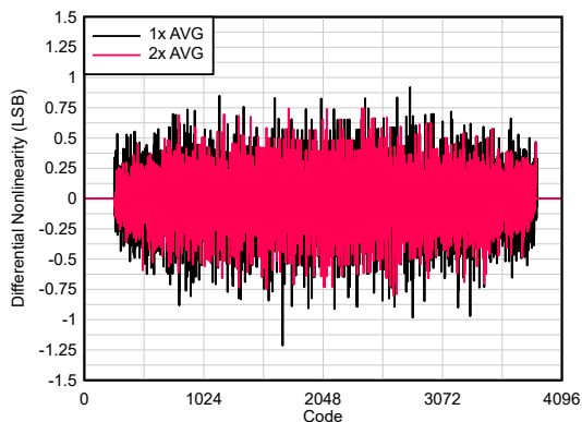
图 5-39. DNL vs Code
