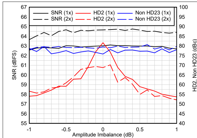
图 6-3. Amplitude Imbalance - 2.6 GSPS
