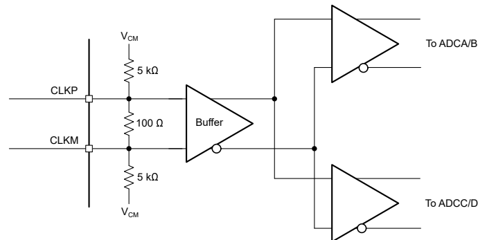
图 6-14. Clock Input Internal Circuitry
