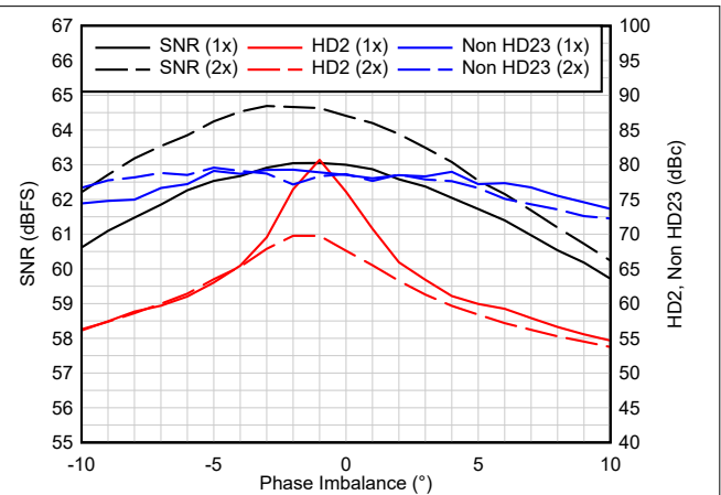
图 6-4. Phase Imbalance - 2.6 GSPS
