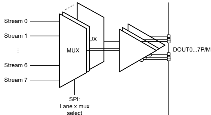
图 6-43. SERDES output mux for DOUT0
