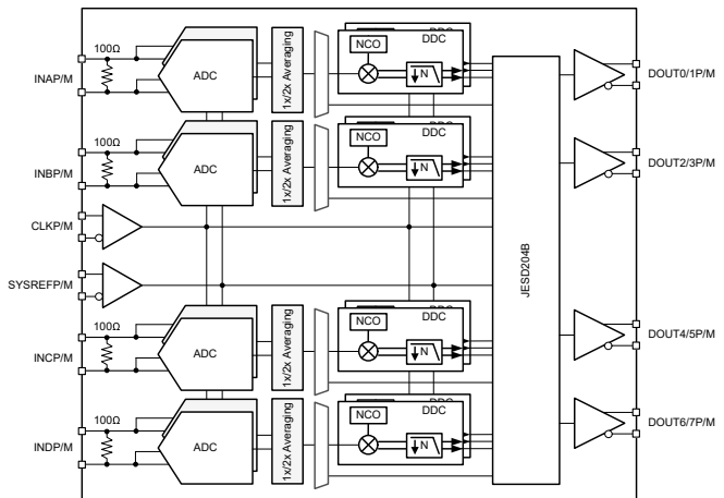
方框图
