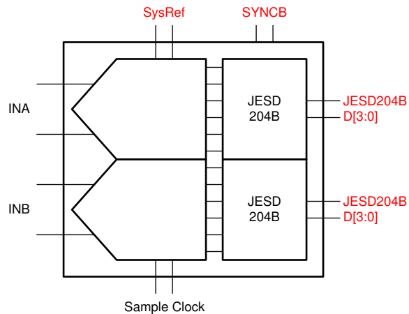
图 8-53. JESD Signal Overview
