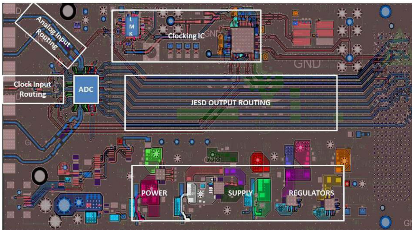
图 11-1. ADC32RF8xEVM Layout
