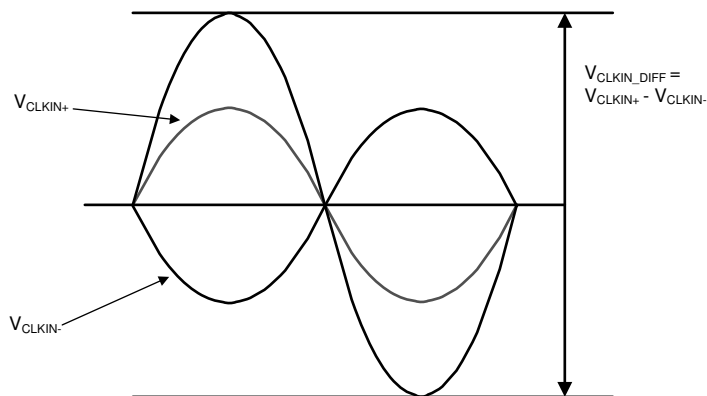
图 7-1. Input Clock Diagram
