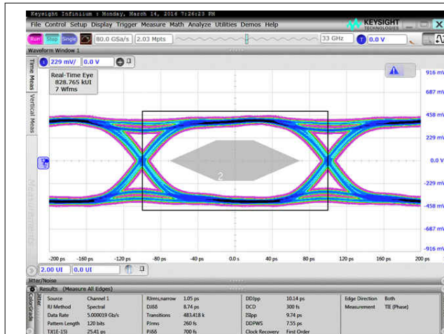
图 8-44. Data Eye at 5 Gbps
