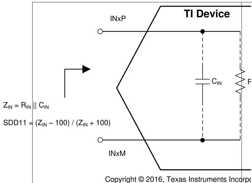
图 8-1. Equivalent Input Impedance
