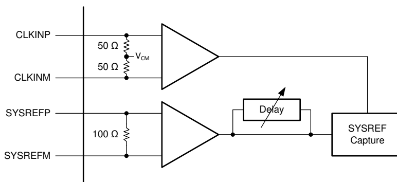
图 8-10. SYSREF Internal Circuit Diagram
