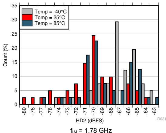
图 6-55. HD2 Histogram at AVDD19 = 1.8 V
