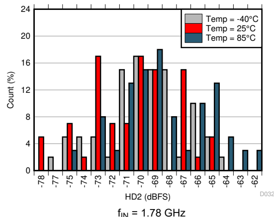
图 6-56. HD2 Histogram at AVDD19 = 1.9 V
