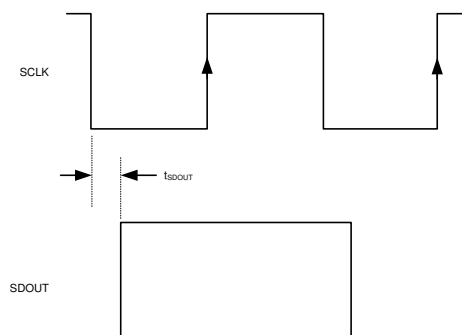
图 8-57. SDOUT Timing
