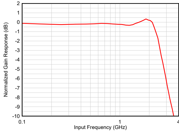
图 7-4. 输入带宽图
