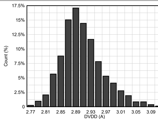
图 6-115. DVDD Distribution
