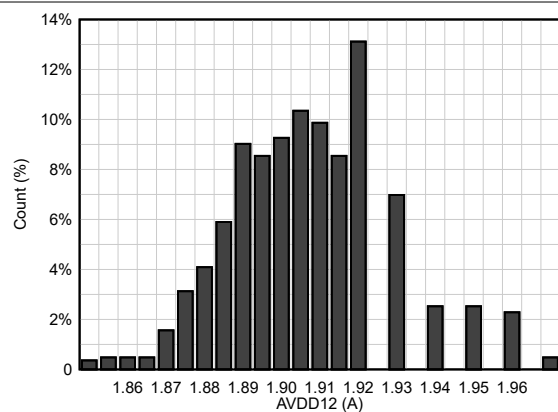
图 6-114. AVDD12 Distribution
