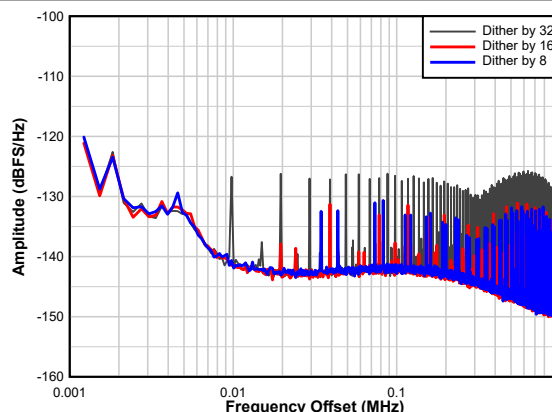
图 7-9. Dither vs Dither Divider Setting
