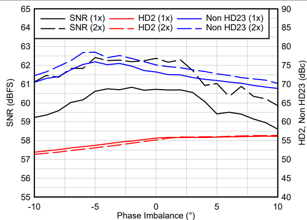
图 7-6. Phase Imbalance - 3.0 GSPS
