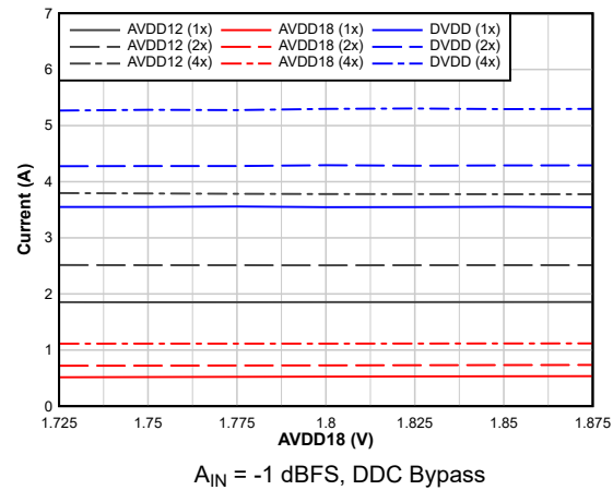
图 6-110. I_{AVDD18} vs Supply
