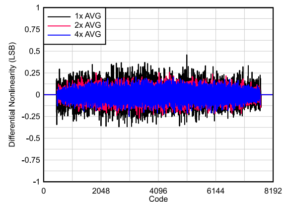
图 6-44. DNL vs Code
