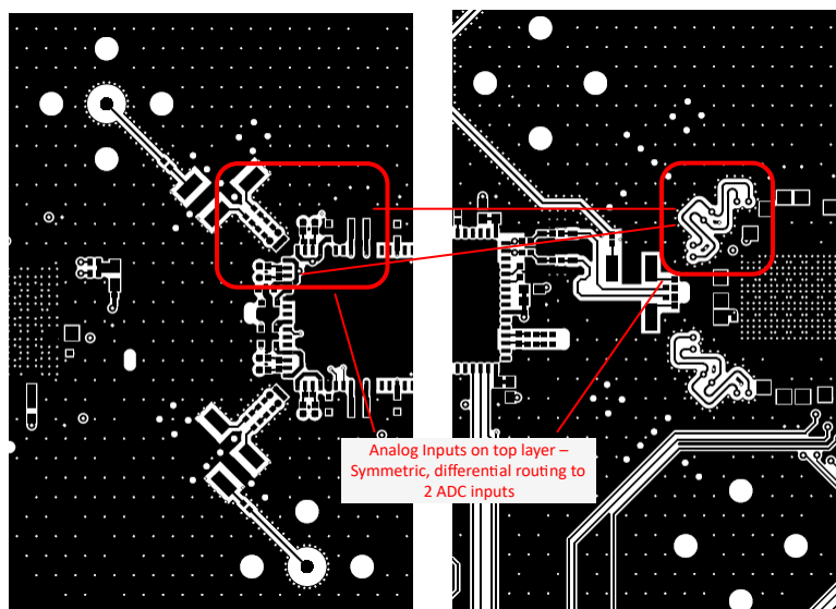
图 8-8. Layout example for 4x AVG: ADC32RF5x EVM
