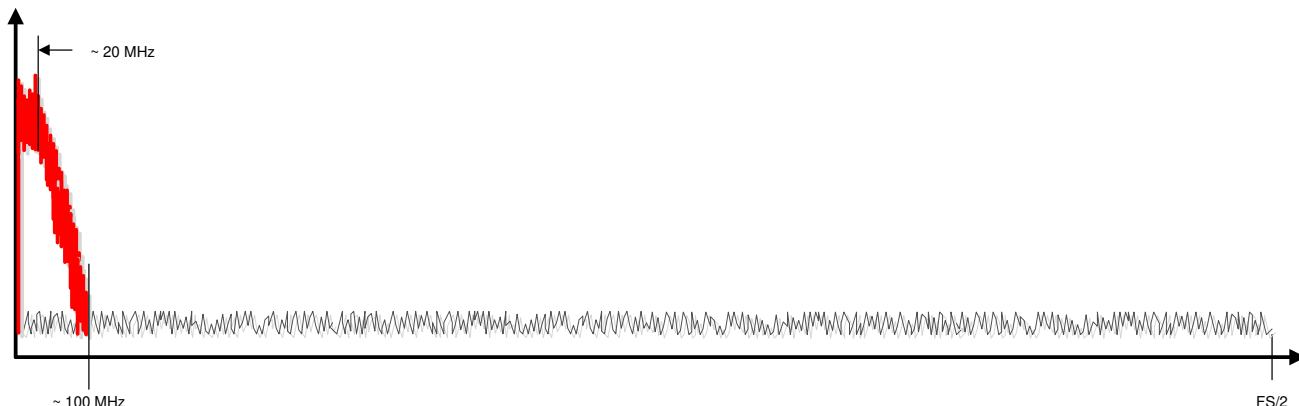
图 7-7. Analog out-of-band dither
