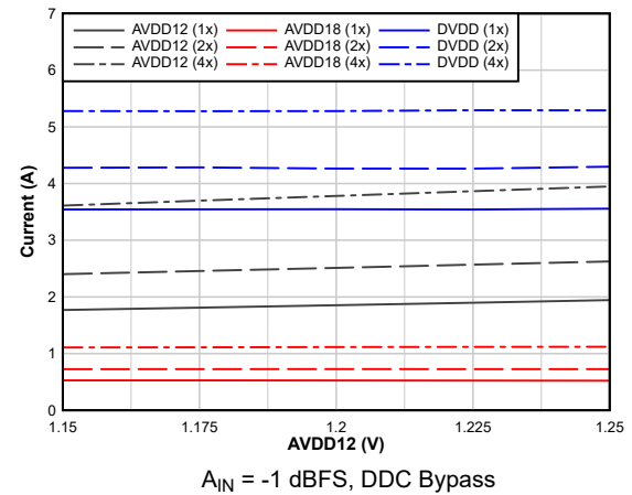
图 6-111. I_{AVDD12} vs Supply
