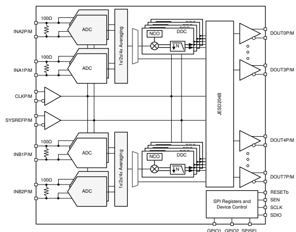
方框图
