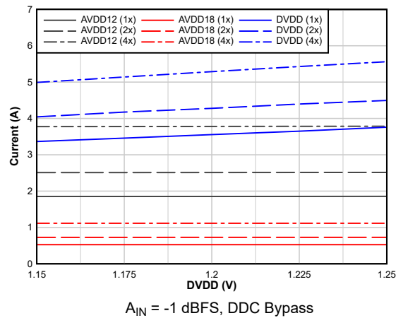
图 6-112. I_{DVDD} vs Supply
