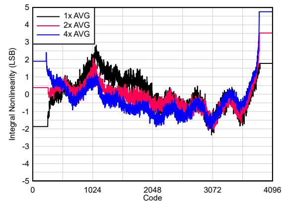
图 6-97. INL vs Code
