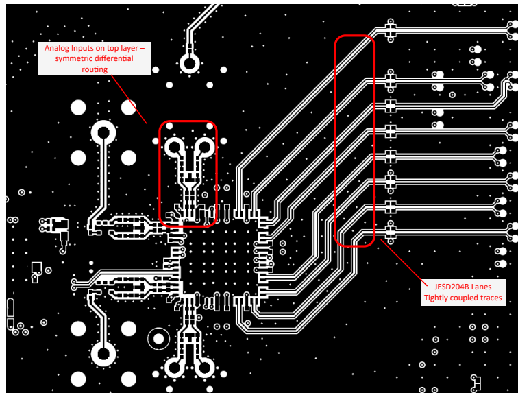
图 8-7. Layout example: top layer of ADC32RF5x EVM
