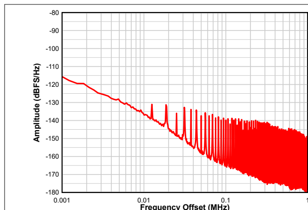
图 7-8. Dither Close-Up
