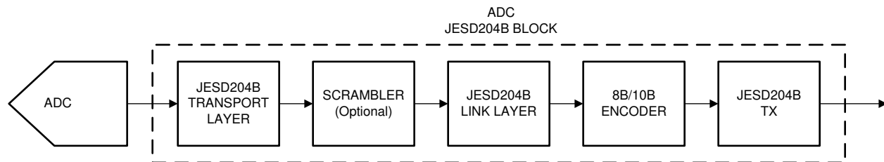
图 7-41. JESD204B Block Diagram
