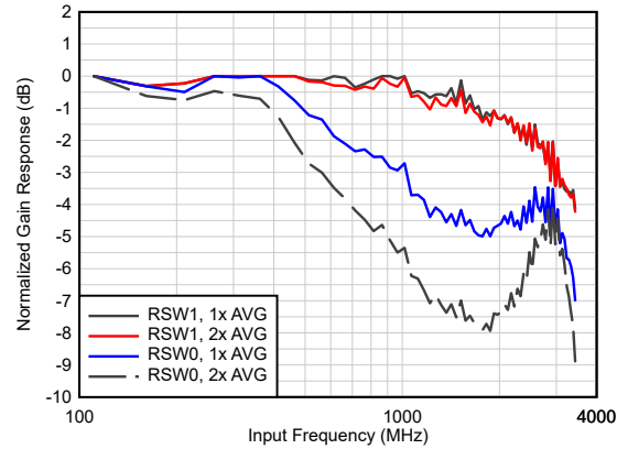
图 7-2. Input Bandwidth - Reset switch DIS
