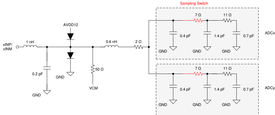
图 7-1. Equivalent Input Schematic
