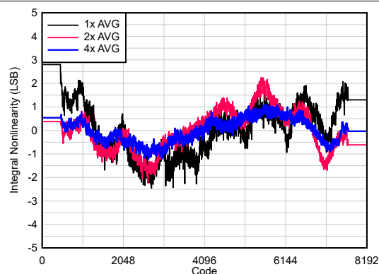
图 6-44. INL vs Code
