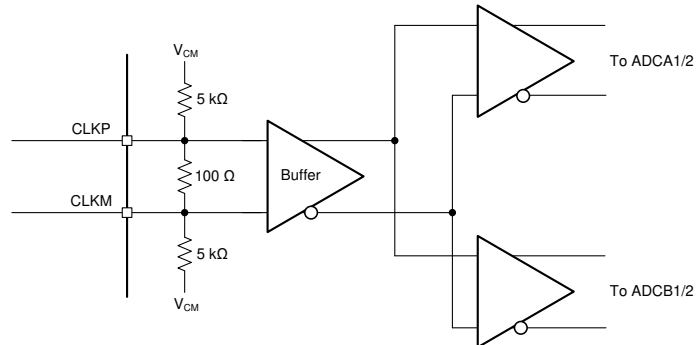
图 7-11. Clock Input Internal Circuitry
