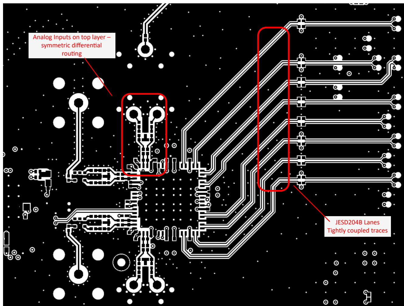
图 8-7. Layout example: top layer of ADC32RF5x EVM
