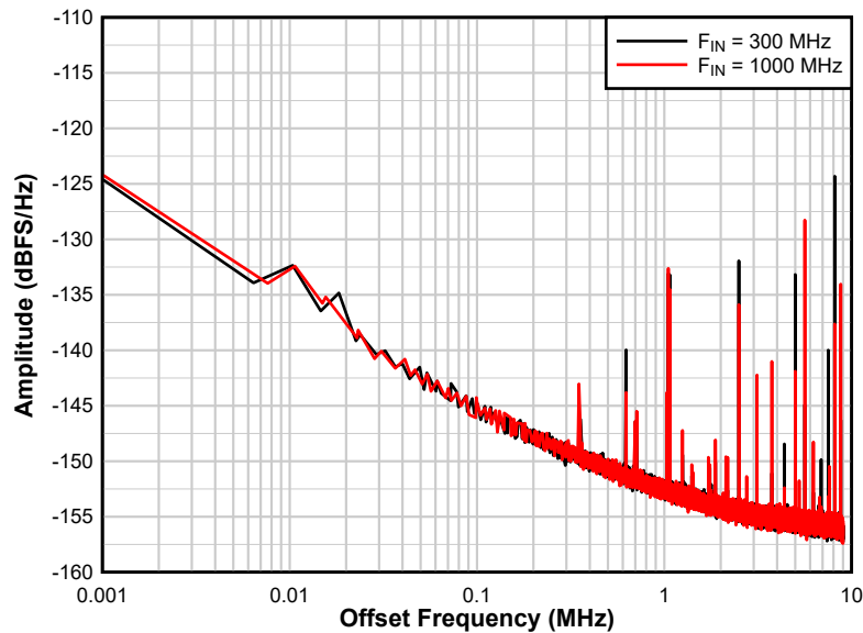
图 7-8. Amplitude Noise
