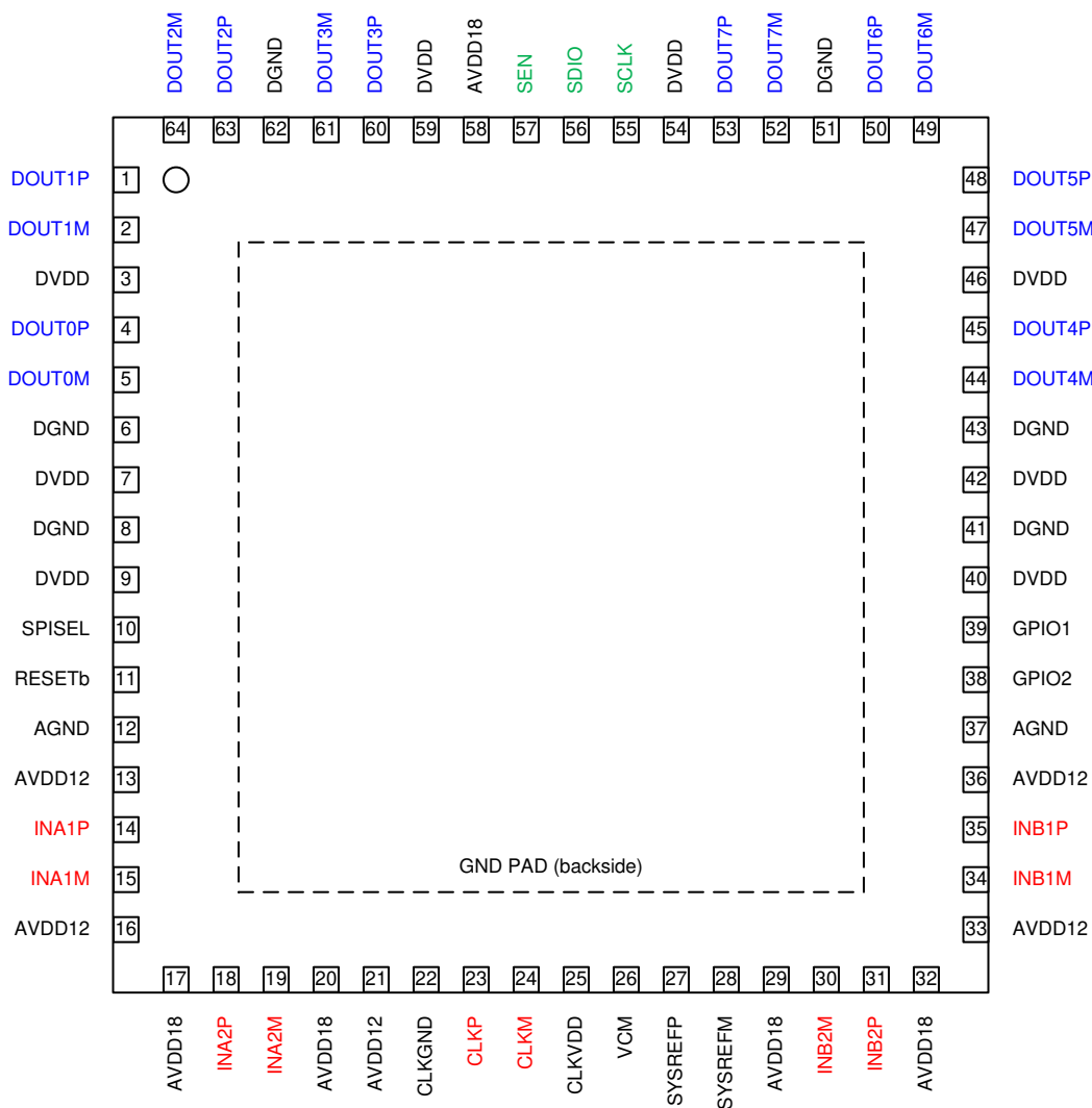
图 5-1. RTD (VQFN) Package, 64 Pin (Top View)
