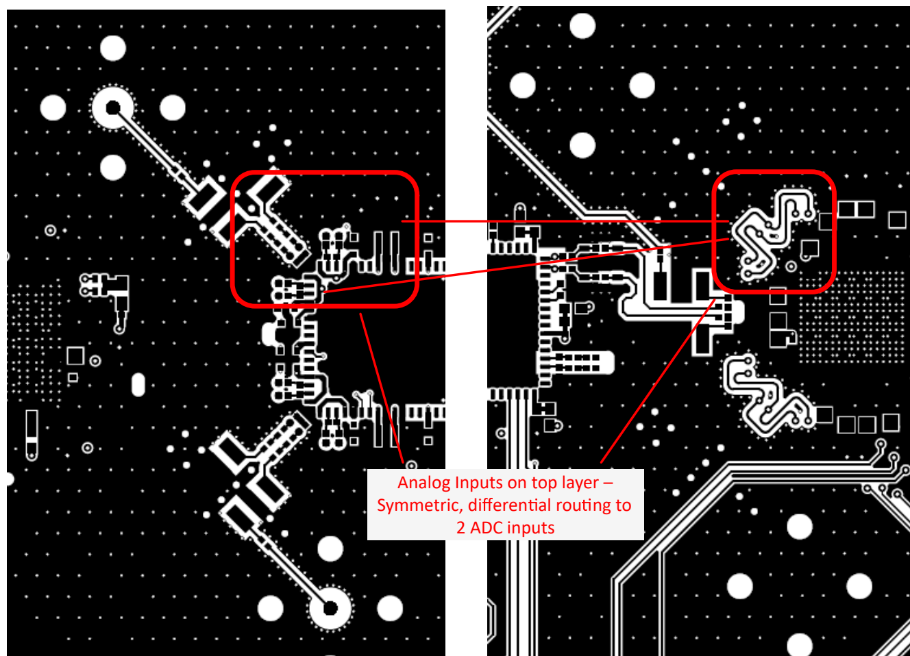
图 8-8. Layout example for 4x AVG: ADC32RF5x EVM
