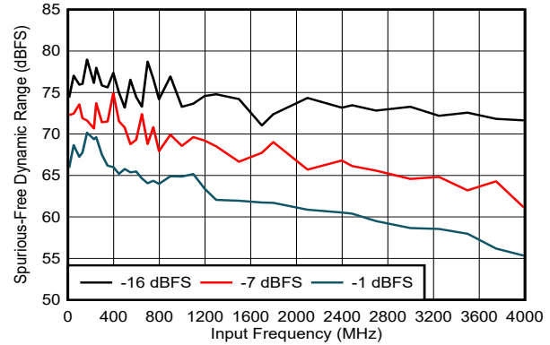
图 5-187. SFDR vs Input Frequency
