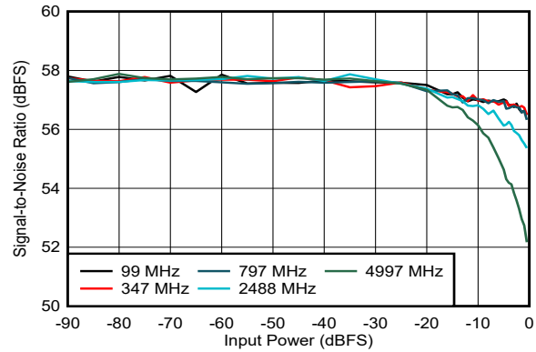
图 5-231. SNR vs Input Power
