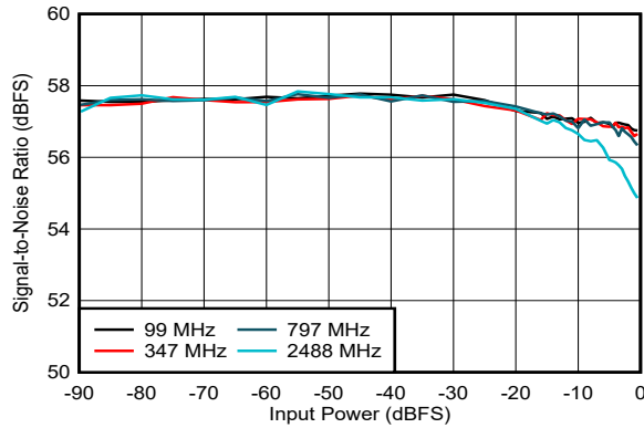
图 5-230. SNR vs Input Power
