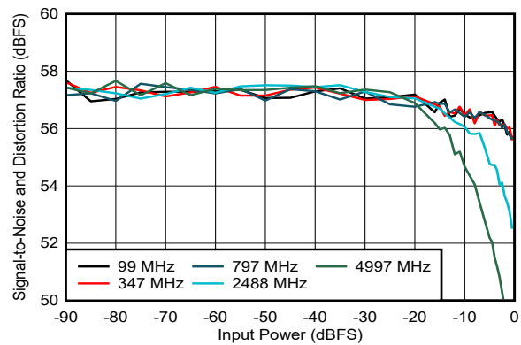
图 5-231. SNR vs Input Power
