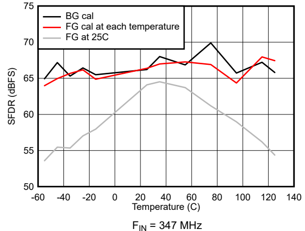
图 5-44. SFDR vs Temperature
