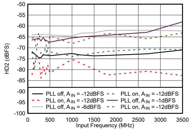
图 5-24. HD2 vs Input Frequency
