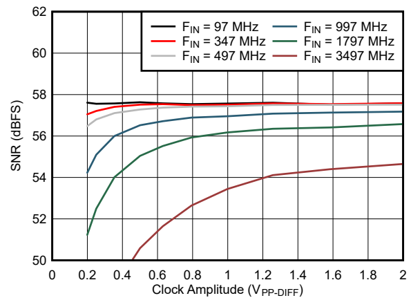
图 5-40. SNR vs Clock Amplitude
