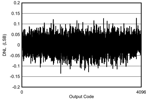
图 5-1. DNL vs Code
