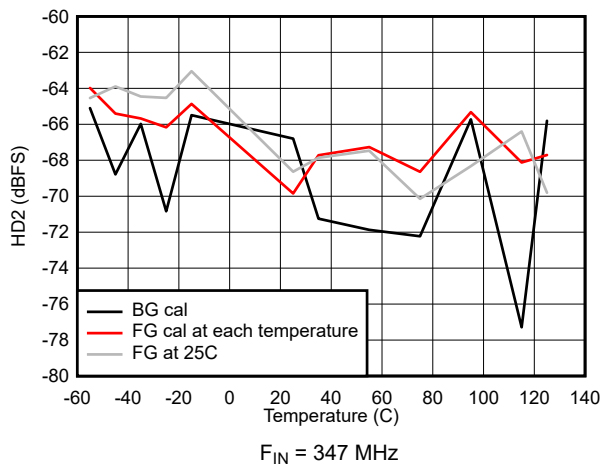
图 5-45. HD2 vs Temperature
