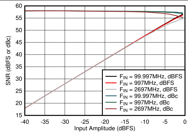
图 5-32. SNR vs Input Amplitude
