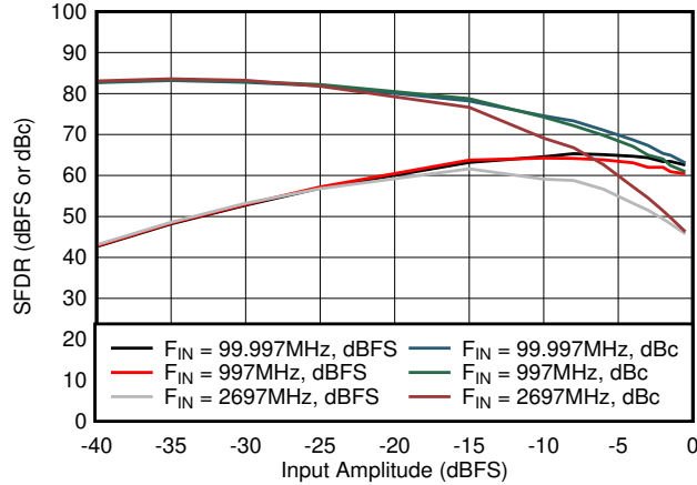
图 5-33. SFDR vs Input Amplitude
