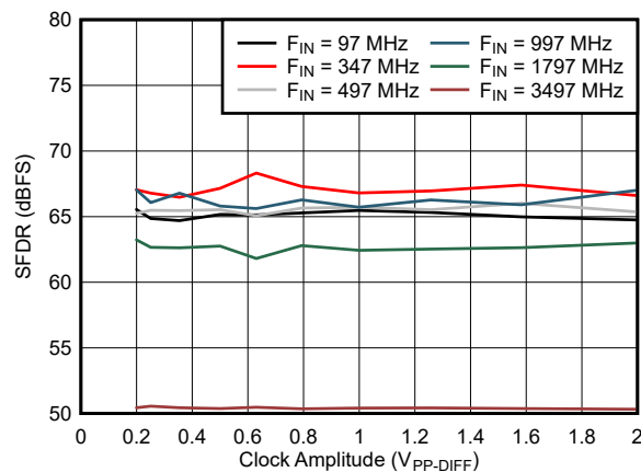
图 5-41. SFDR vs Clock Amplitude
