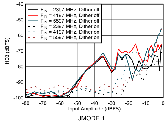
图 5-18. DES Mode: HD3 vs Input Amplitude
