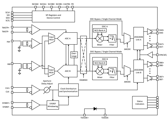
ADC12DJ5200SE 方框图
