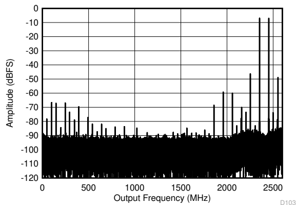
图 5-26. 双通道模式：4197MHz 时的双音 FFT
