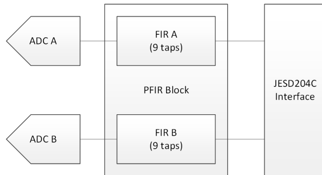
图 6-4. 双通道均衡 PFIR 方框图
