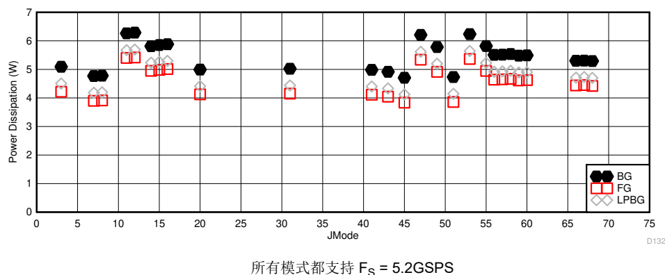
图 5-118. 双通道模式：在 5.2GSPS 时的功率与 JMODE 间的关系
