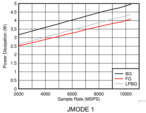
图 5-129. DES 模式：功耗与采样率间的关系
