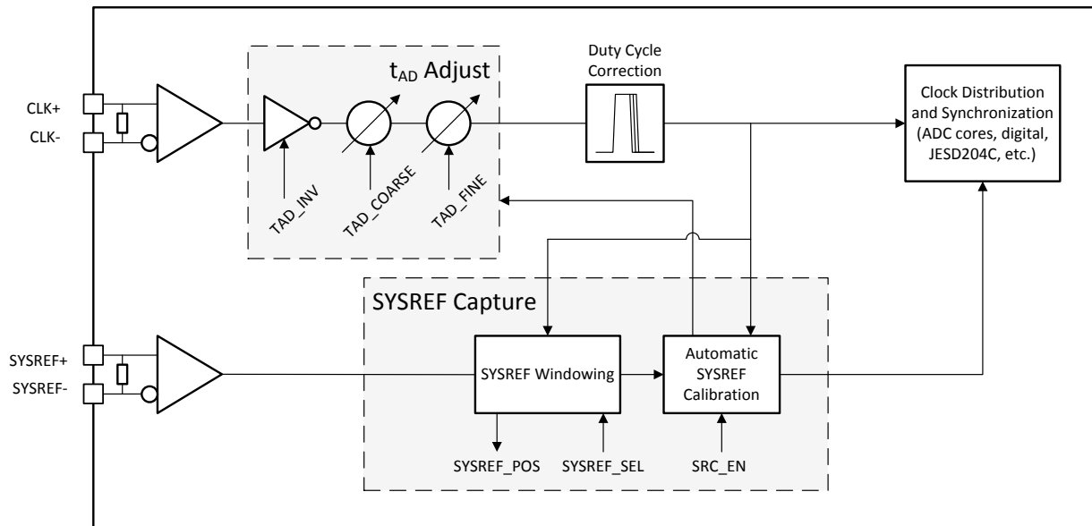
图 7-2. Clocking Subsystem
