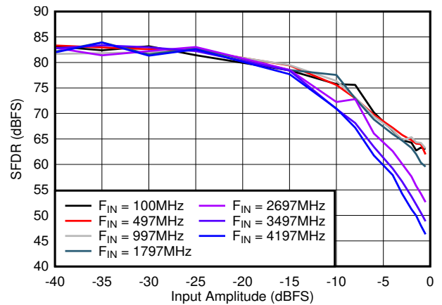
图 6-32. SFDR vs A_{IN}
