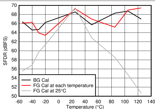
图 6-65. SFDR vs Temperature
