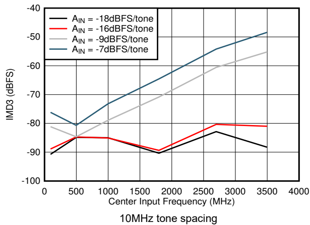
图 6-75. IMD3 vs F_{IN}
