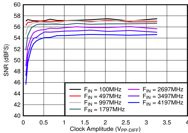
图 6-37. SNR vs A_{CLK}
