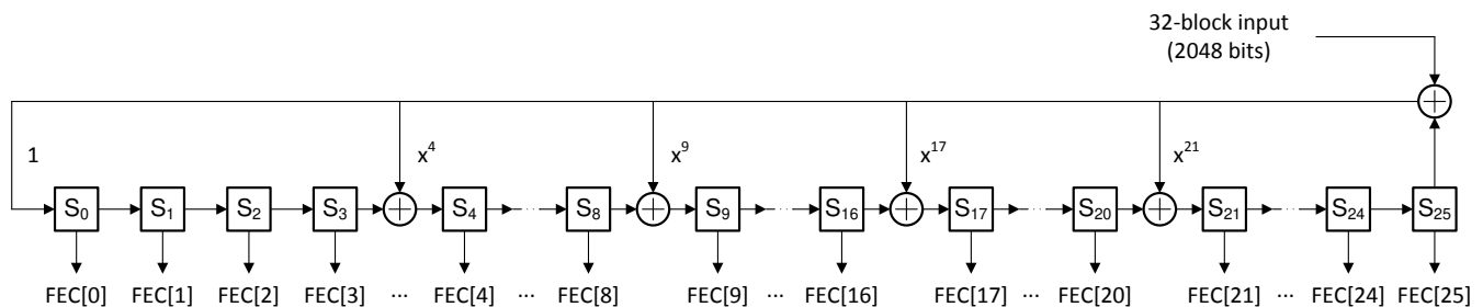
图 7-10. FEC Parity Bit Generator
