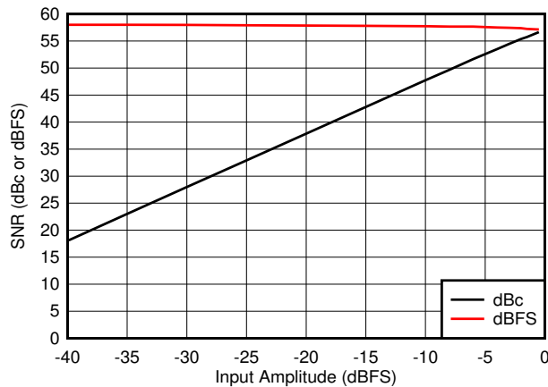
图 6-33. SNR vs A_{IN}
