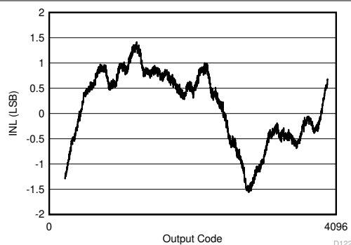
图 6-2. INL vs Code
