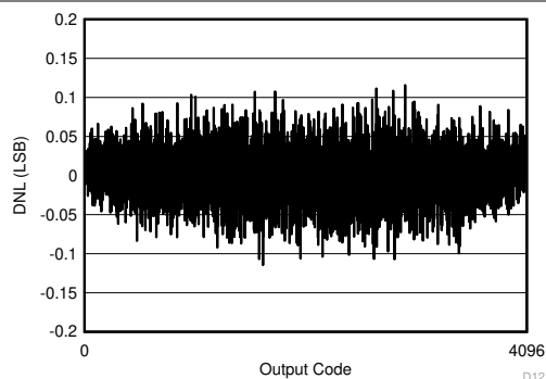
图 6-1. DNL vs Code
