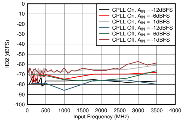
图 6-52. HD2 vs A_{IN} and C-PLL
