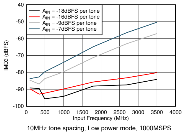
图 6-76. IMD3 vs F_{IN}
