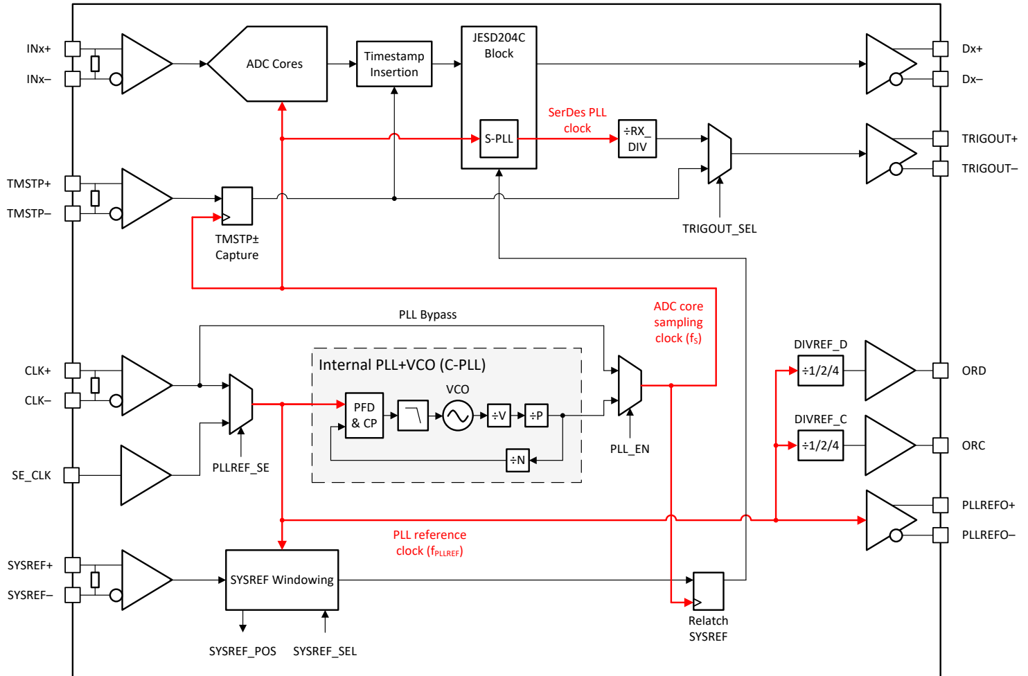
图 7-5. Clocking Subsystem
