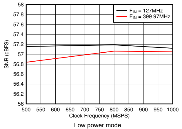
图 6-28. SNR vs Sample Rate
