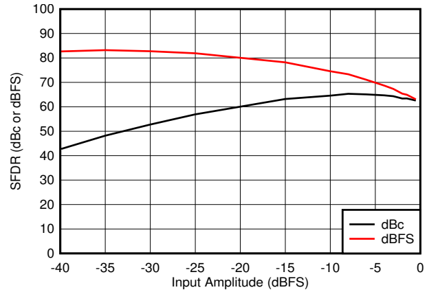
图 6-34. SFDR vs A_{IN}
