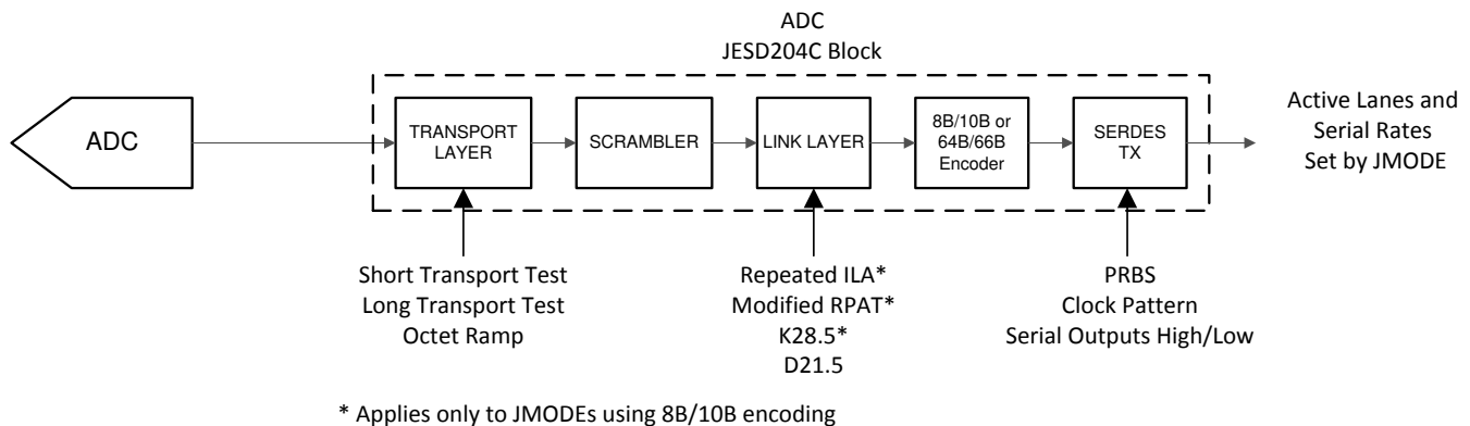
图 7-14. Test Mode Insertion Points
