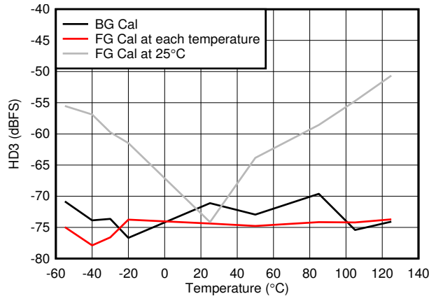
图 6-67. HD3 vs Temperature
