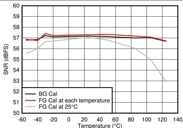
图 6-64. SNR vs Temperature
