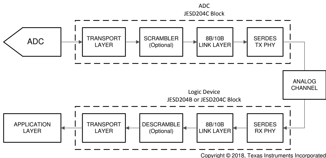
图 7-7. Simplified 8B/10B Encoded JESD204C Interface Diagram
