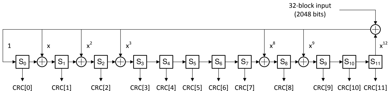
图 7-9. CRC-12 Parity Bit Generator
