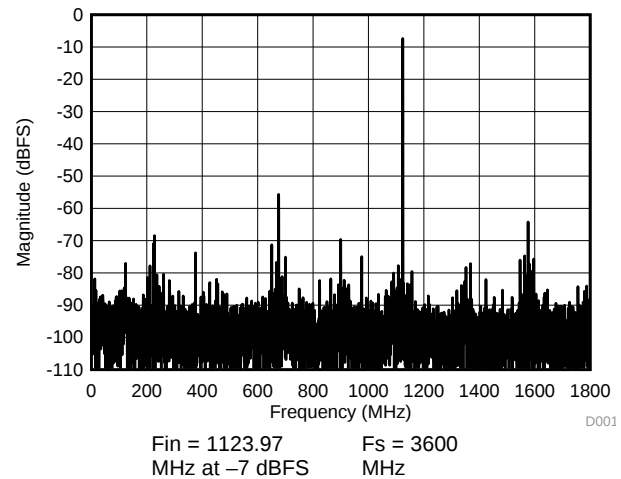
Figure 6-9. Spectrum DES Mode
