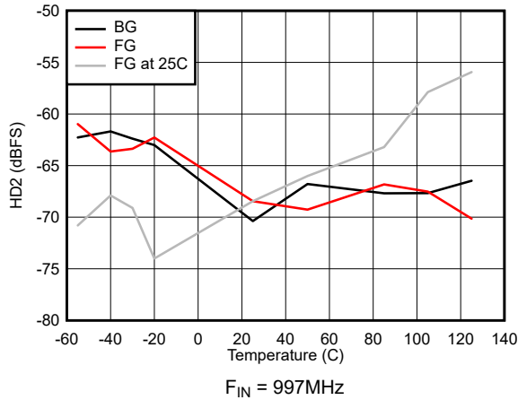
图 5-37. HD2 vs Temperature
