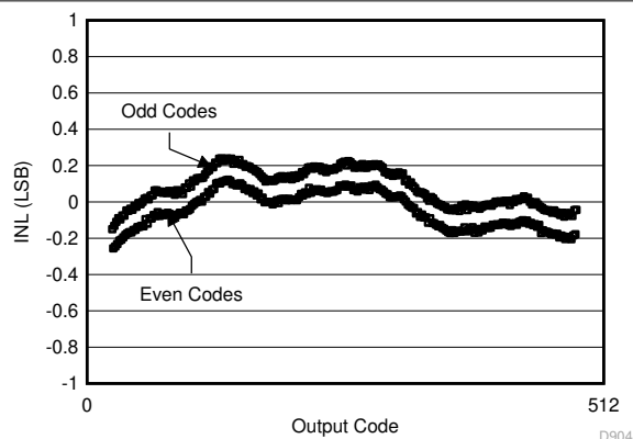
图 5-2. INL vs Code
