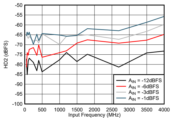
图 5-18. HD2 vs Input Frequency
