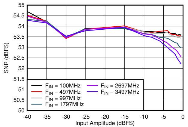
图 5-30. SNR vs Input Amplitude
