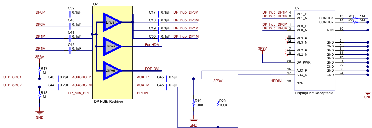
图 45. DisplayPort Implementation
