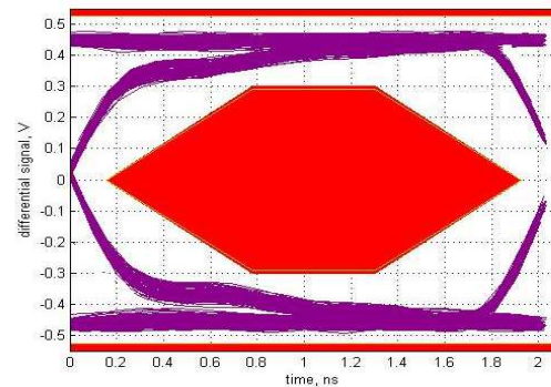
图 39. Downstream Port 3
