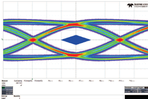
图 38. Downstream Port 2
