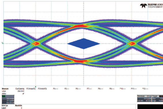
图 36. Upstream Port
