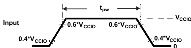
图 7-8. FlexRay Inputs
