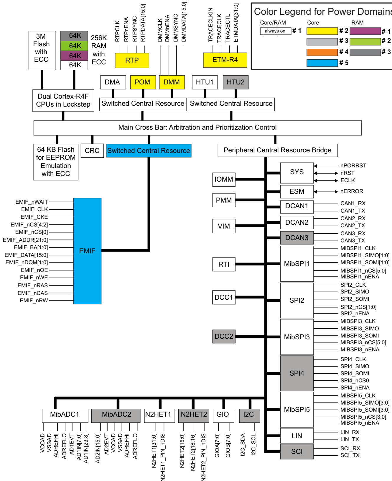
图 1-1. 功能方框图
