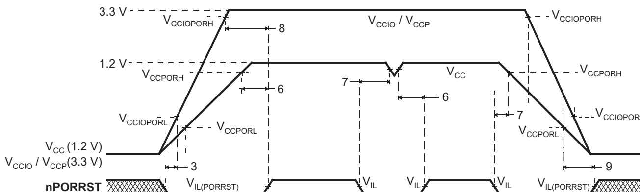
图 5-1. nPORRST 时序图
