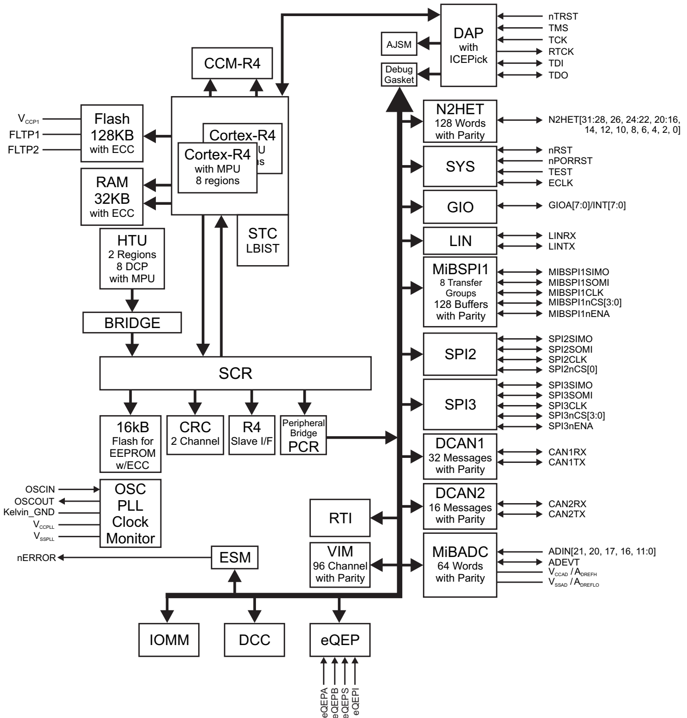
图 1-1. 功能方框图
