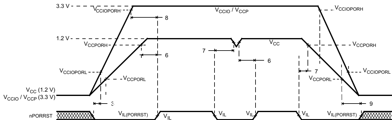
图 7-1. nPORRST Timing Diagram (A)
