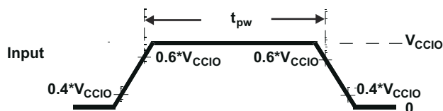
图 6-4. FlexRay Inputs
