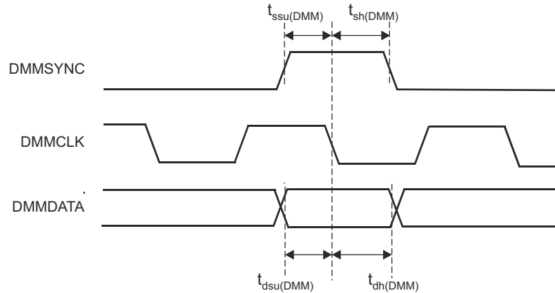
图 7-36. DMMDATA Timing
