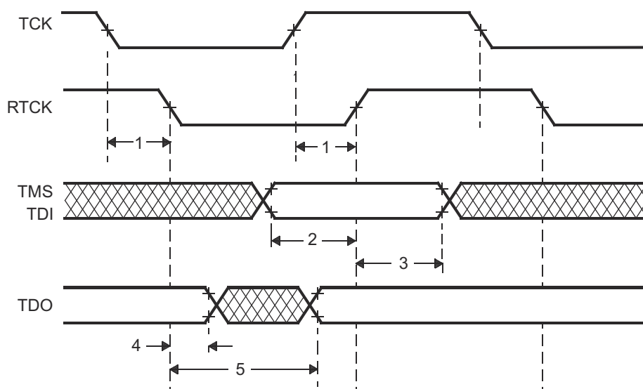
图 7-28. JTAG Timing
