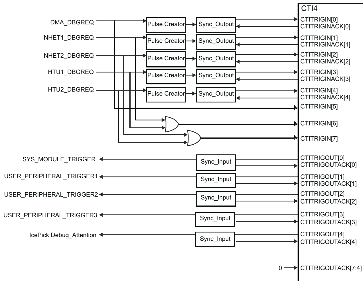
图 7-27. CTI4 Mapping
