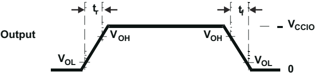
图 6-5. CMOS-Level Outputs
