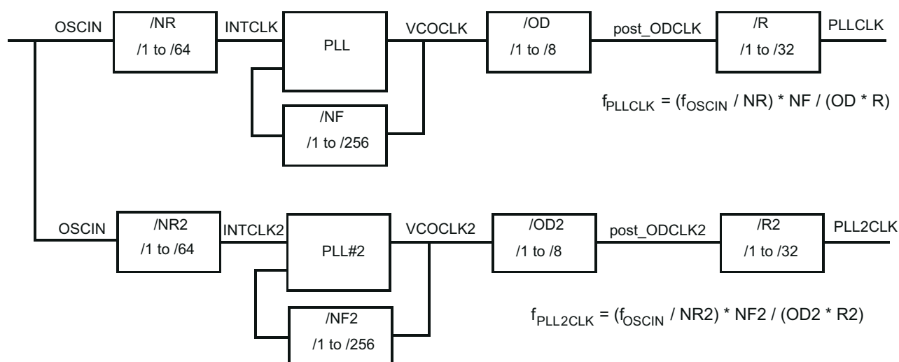
图 7-5. GWT PLLx Block Diagram
