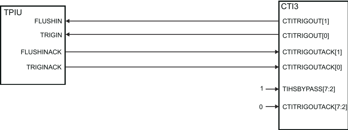
图 7-26. CTI3 Mapping
