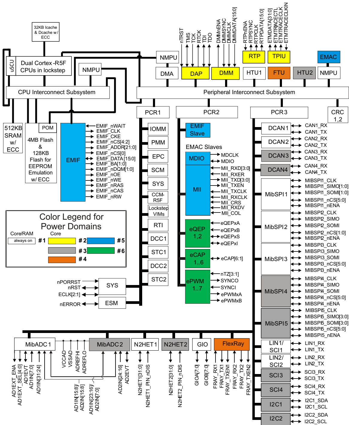
图 1-1. 功能方框图
