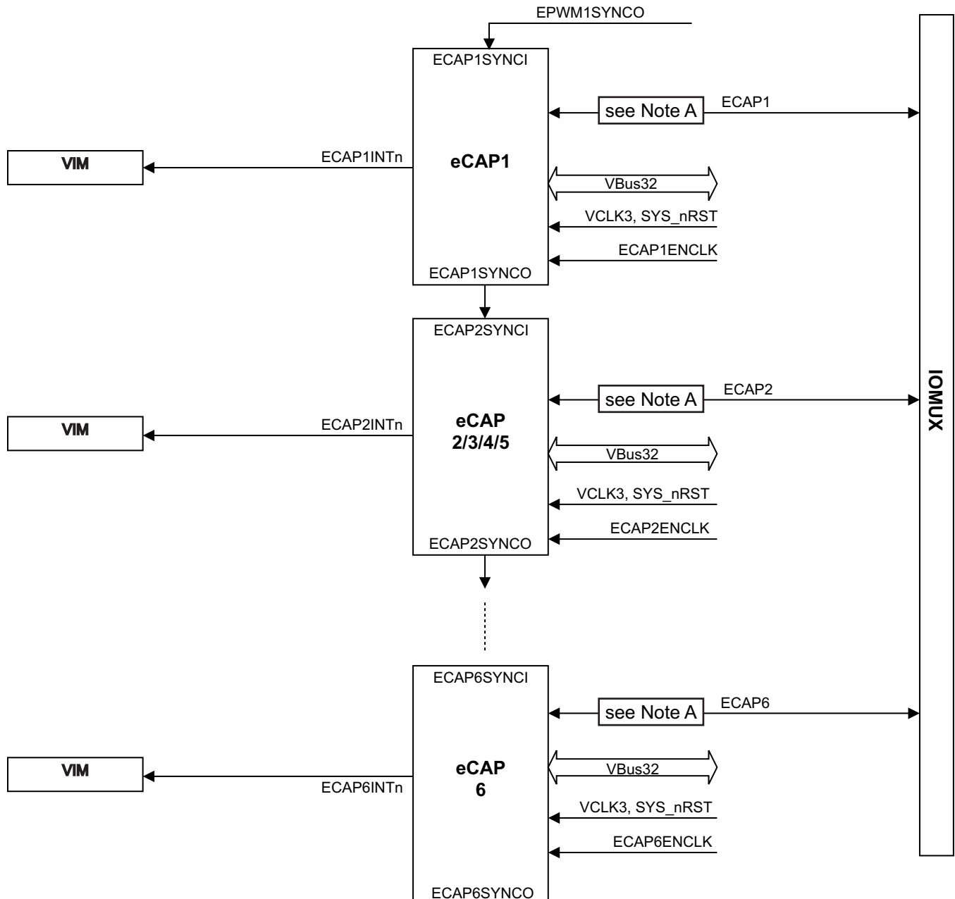
图 7-4. eCAP Module Connections
