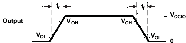
图 5-4. CMOS-Level Outputs
