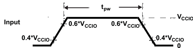
图 5-3. FlexRay Inputs
