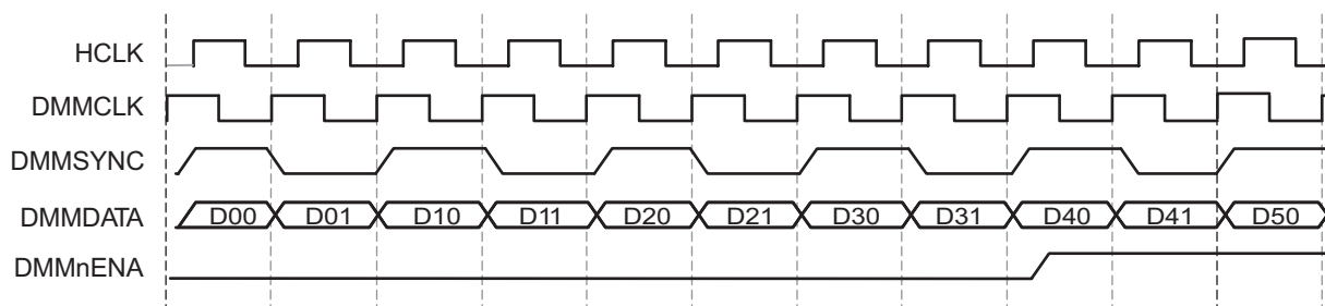
图 6-37. DMMnENA Timing
