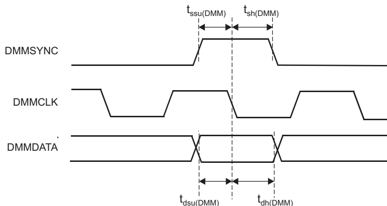
图 6-36. DMMDATA Timing
