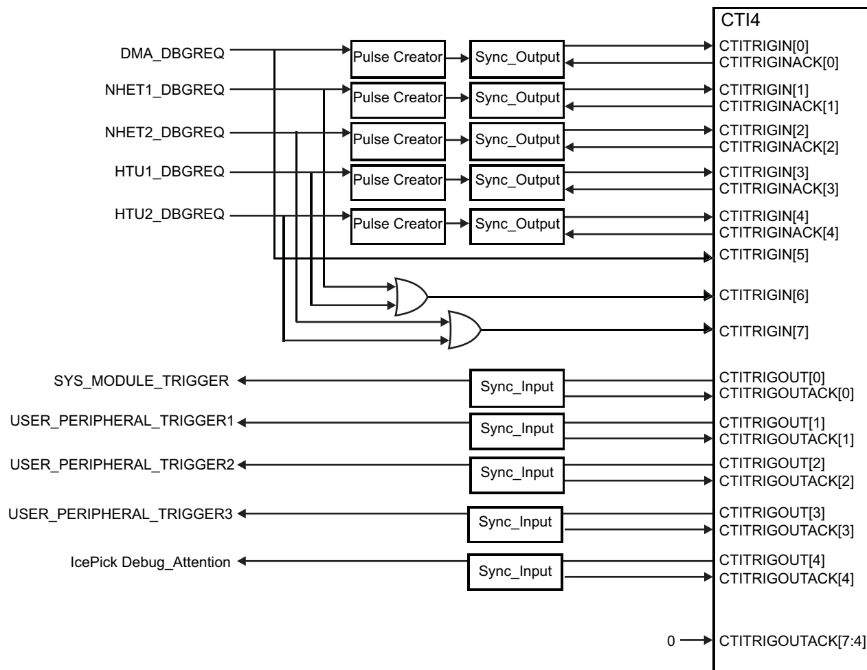
图 6-27. CTI4 Mapping
