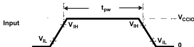
图 5-2. TTL-Level Inputs
