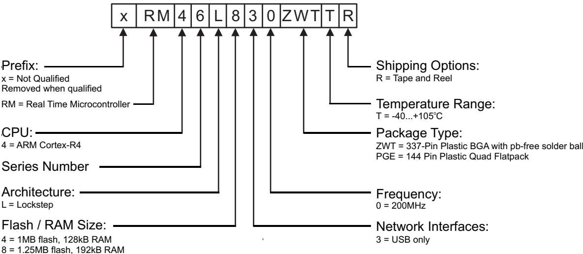
图 7-1. RM46Lx30 器件编号惯例
