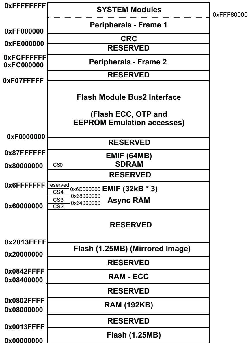
图 5-9. 内存映射
