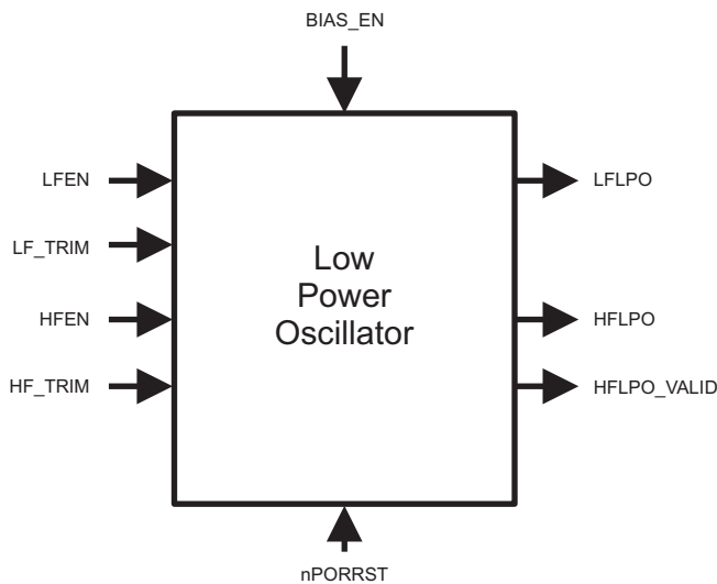
图 5-5. LPO 方框图
