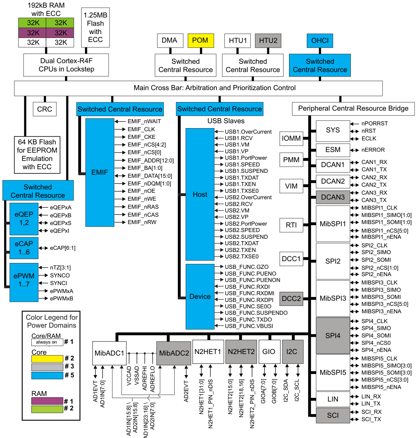
图 1-1. 功能方框图
