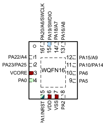
图 6-8. 16 引脚 RTR (WQFN) (顶视图) - MSPM0L130x
