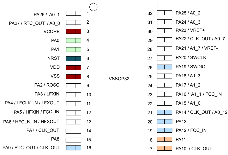
图 6-6. 32 引脚 DGS28 (VSSOP) (顶视图)
