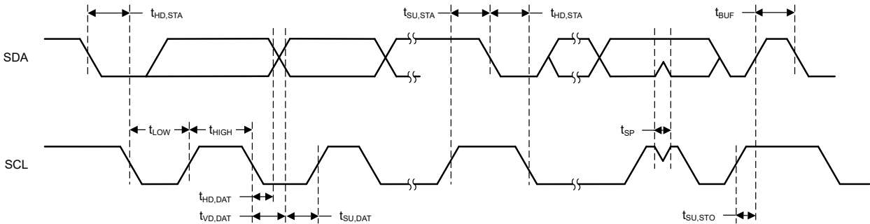
图 7-5. I2C 时序图
