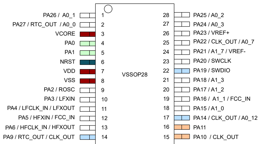
图 6-7. 28 引脚 DGS28 (VSSOP) (顶视图)
