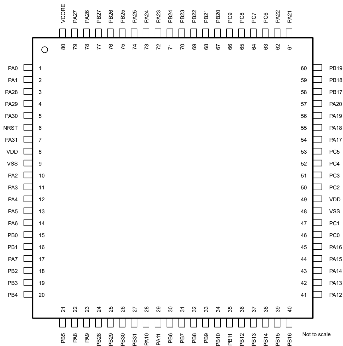
图 6-3. 80 引脚 PN (0.5mm) (LQFP) 封装图
