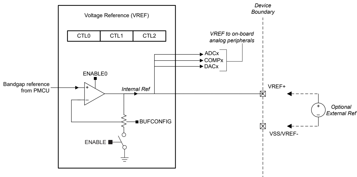
图 8-2. VREF 模块
