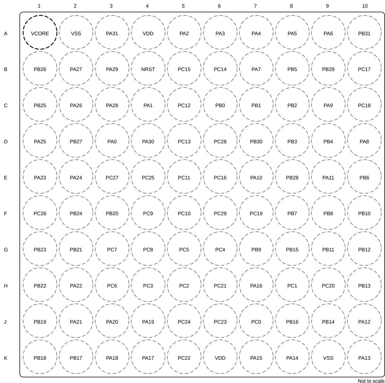
图 6-1. 100 引脚 ZAW (0.8mm) (nFBGA) 封装图
