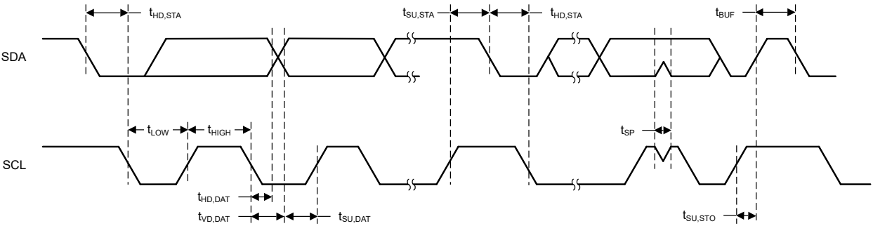
图 7-3. I2C 时序图
