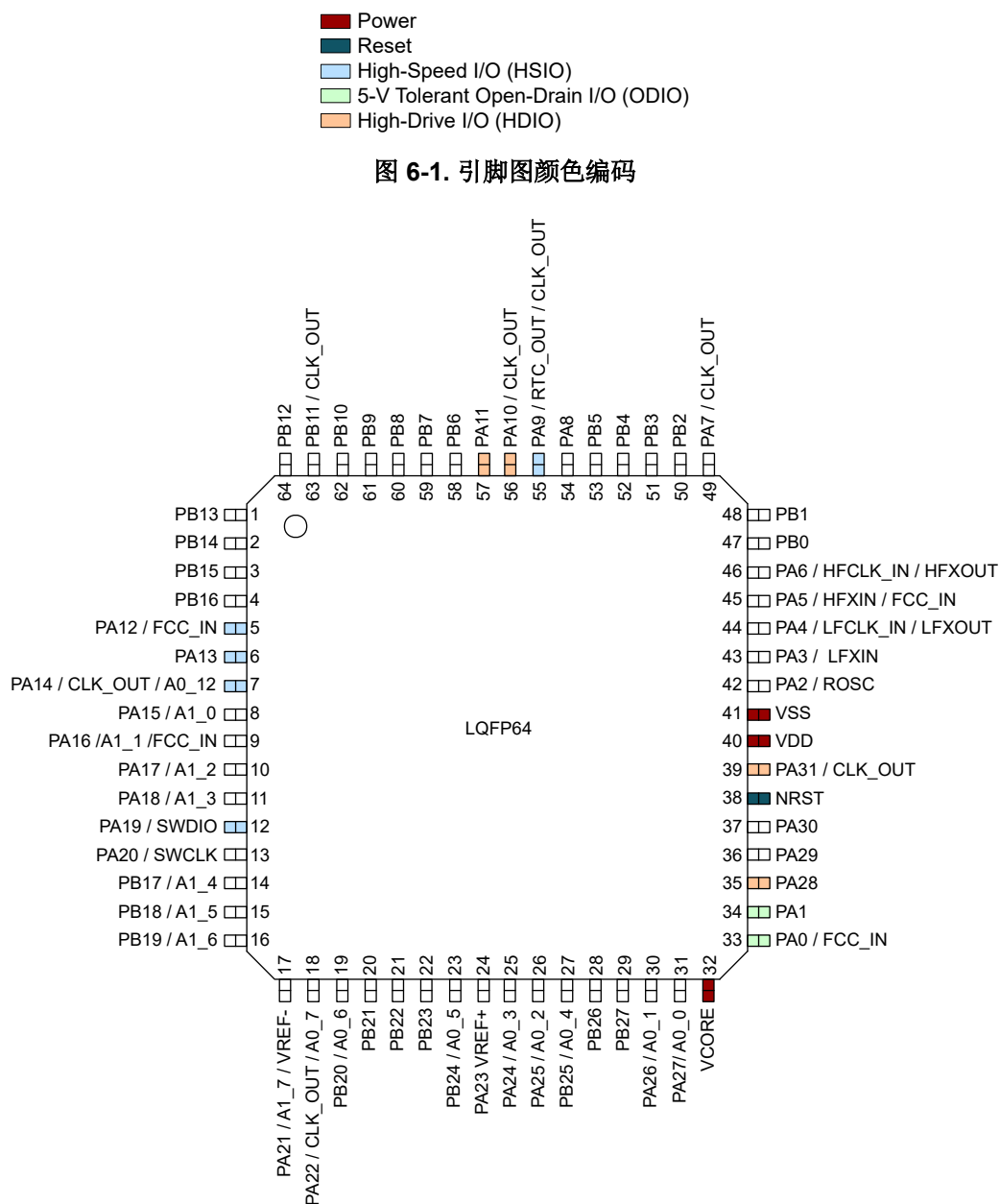
图 6-2. 64 引脚 PM (LQFP) (顶视图)
