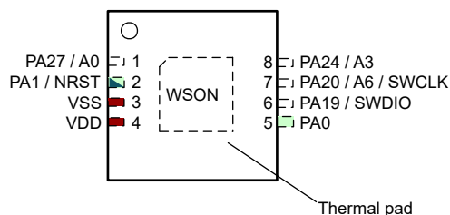
图 6-7. 8-Pin DSG (WSON) (Top View)
