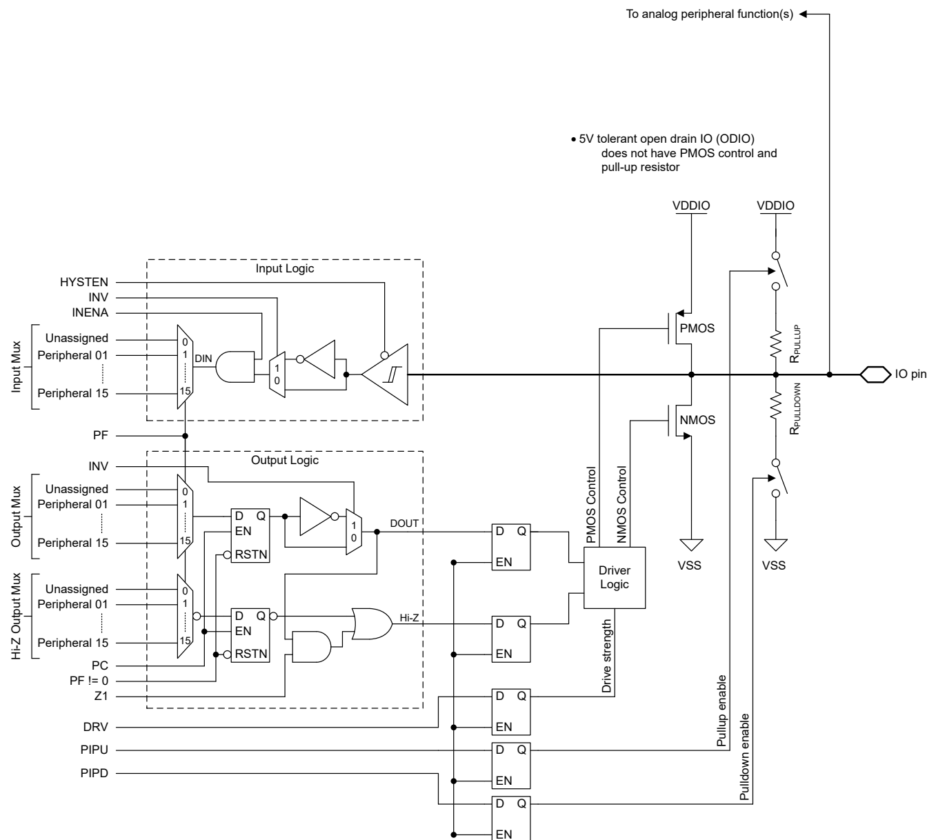
图 8-2. Superset Input/Output Diagram
