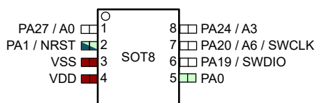
图 6-6. 8-Pin DDF (SOT) (Top View)
