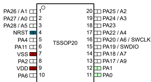
图 6-3. 20-Pin PW20 (TSSOP) (Top View)
