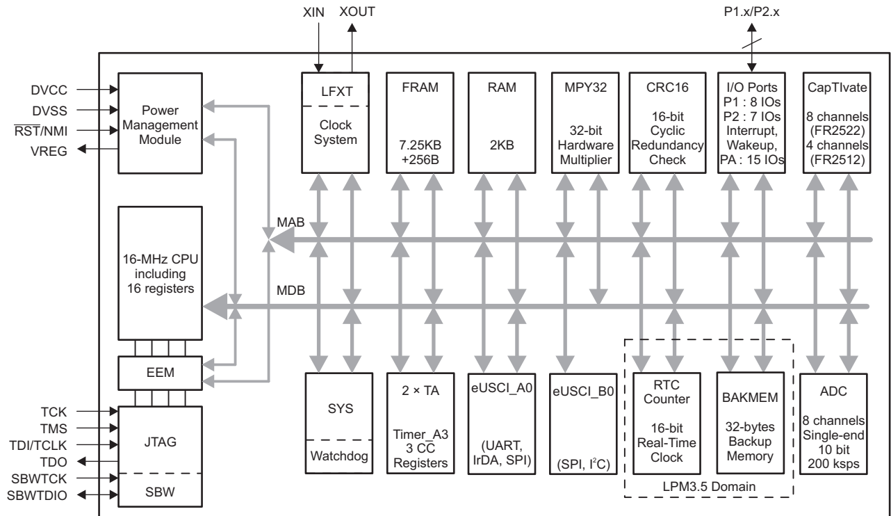
图 1-1. 功能框图
