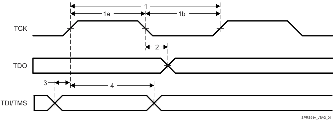
图 6-23. JTAG Timing
