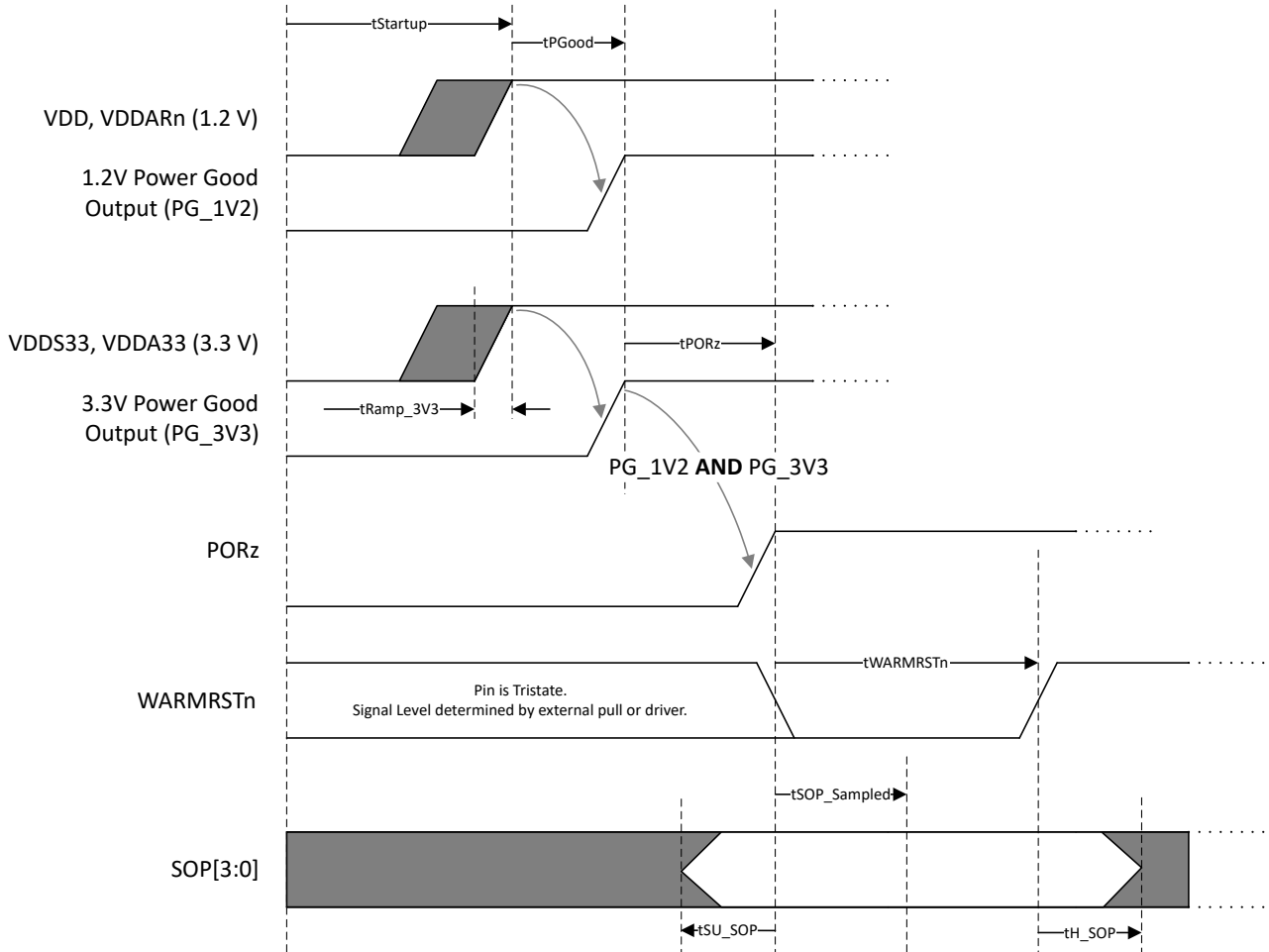
图 6-2. 加电时序
