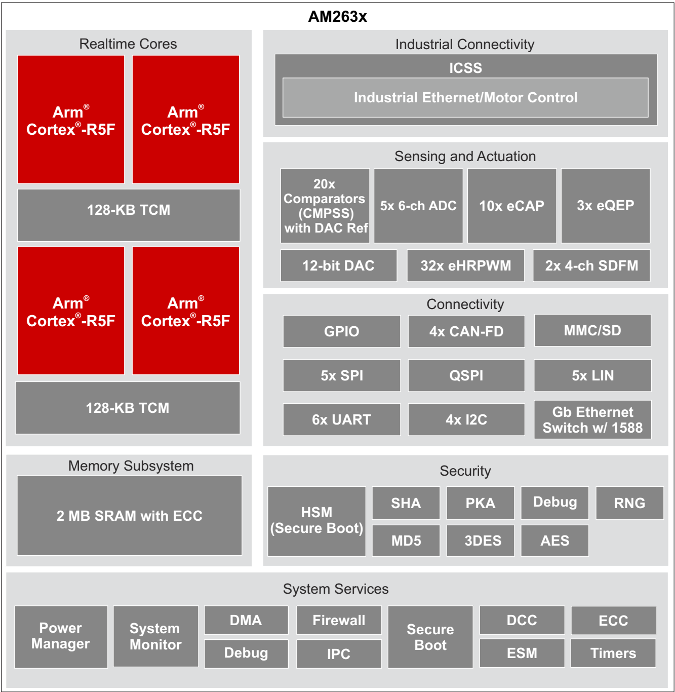
图 3-1. 功能方框图
