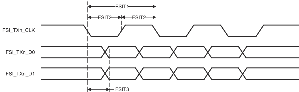
图 6-35. FSI 开关特性 - FSI 模式
