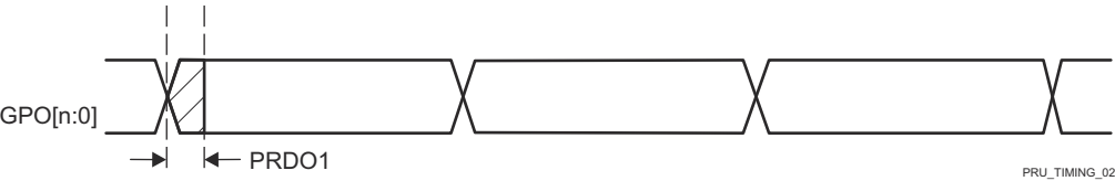
图 6-87. PRU_ICSSG PRU 直接输出时序
