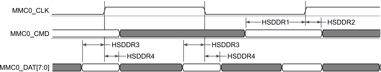
图 6-60. MMC0 - 高速 DDR 模式 - 接收模式
