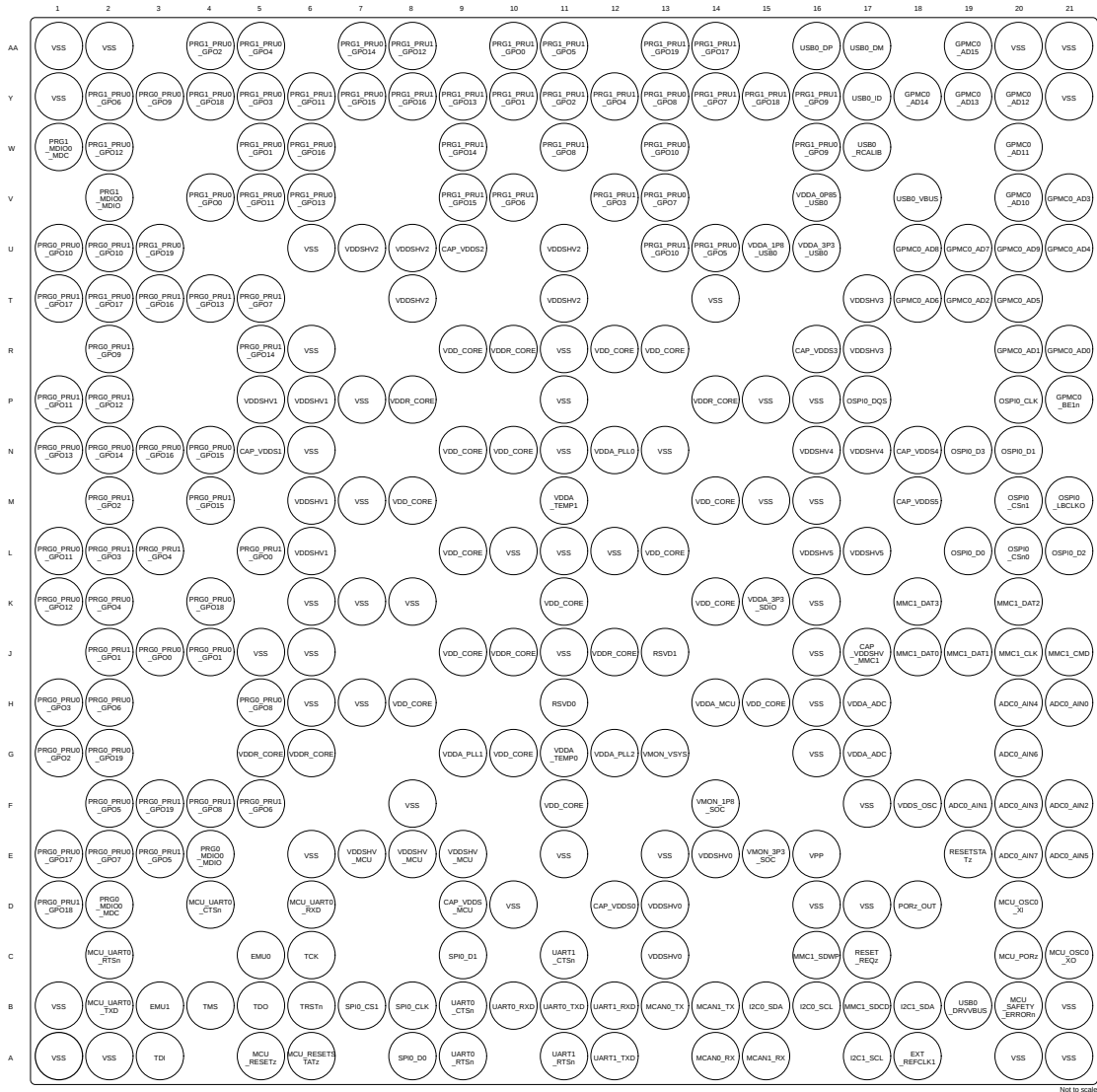
图 5-2. ALX FCBGA-N293 引脚图 (底视图)
