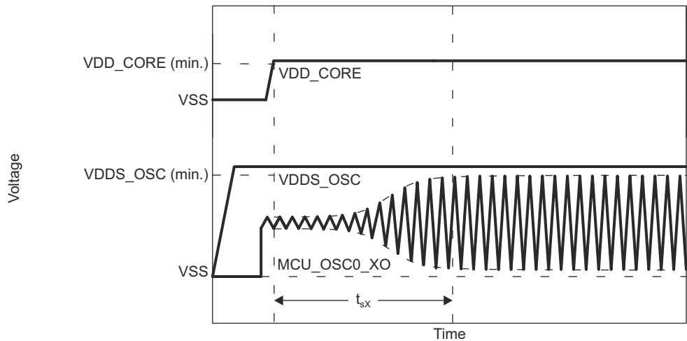
图 6-16. MCU_OSC0 启动时间
