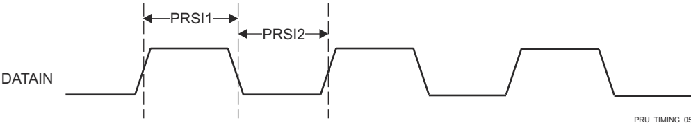
图 6-90. PRU_ICSSG PRU 移入时序
