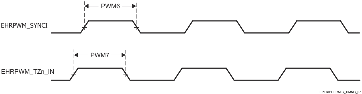
图 6-29. EPWM 时序要求
