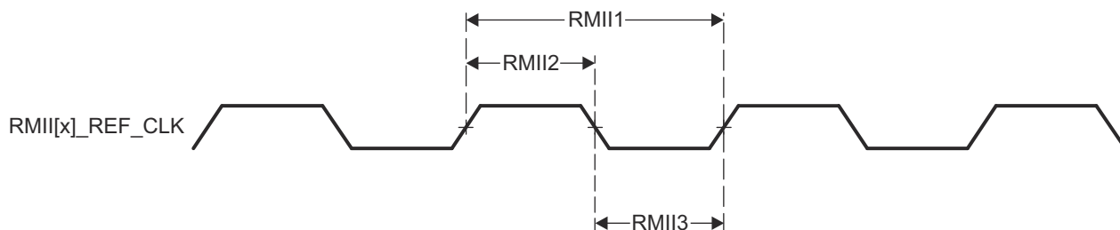
图 6-21. CPSW3G RMII[x]_REF_CLK 时序要求 - RMII 模式
