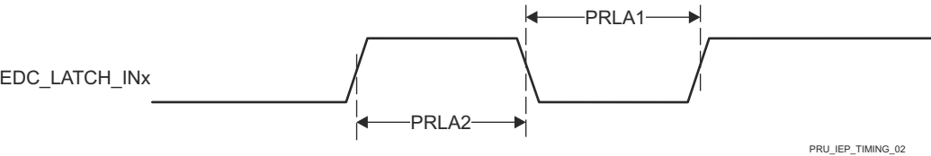
图 6-99. PRU_ICSSG IEP LATCH_INx 时序要求
