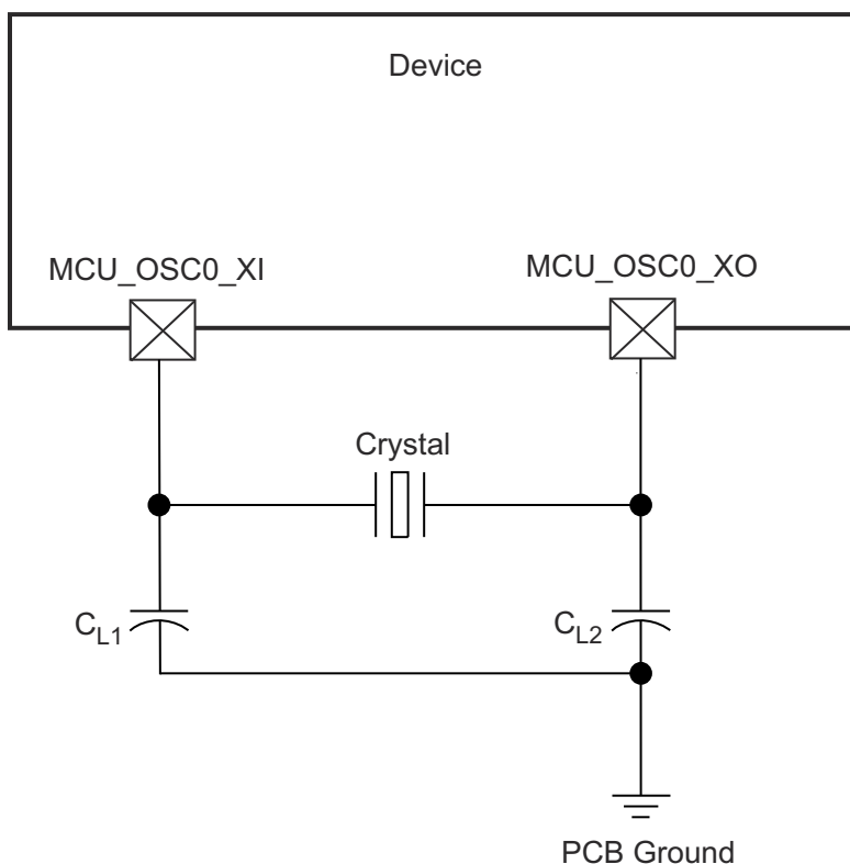
图 6-15. MCU_OSC0 晶体实现
