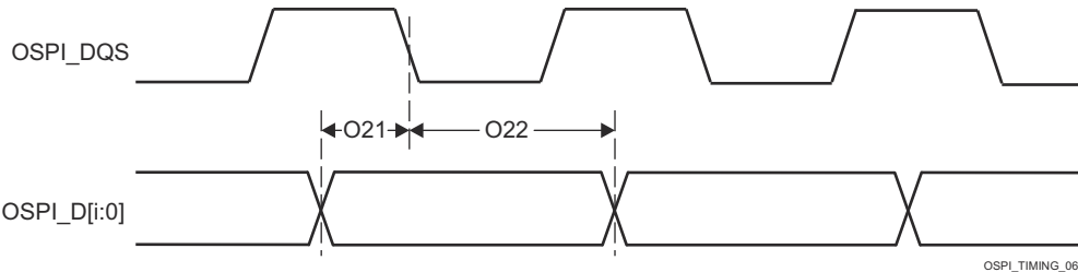
图 6-79. OSPI0 时序要求 - 具有外部电路板环回的 PHY SDR
