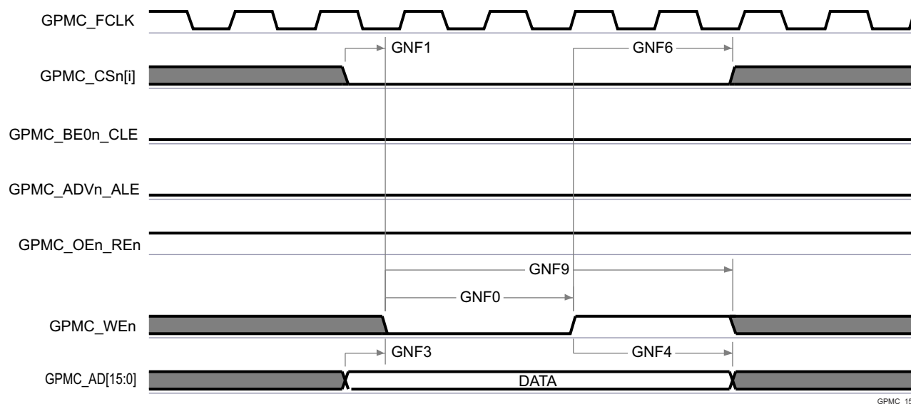
图 6-51. GPMC 和 NAND 闪存 - 数据写入周期
