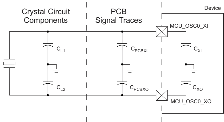
图 6-17. 负载电容
