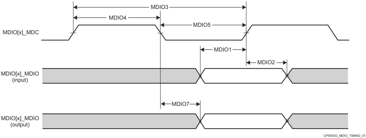
图 6-103. PRU_ICSSG MDIO 时序要求和开关特性
